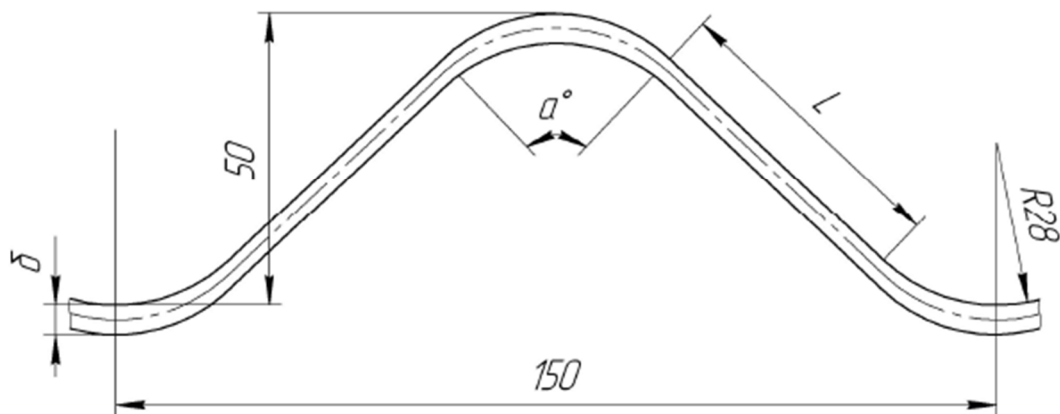
Рисунок 4.1 – Геометрические характеристики профиля КТЦ СМКГ 150x50 мм
