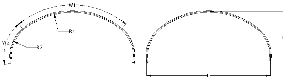
Рисунок 5.13 - Арочные полицентрические низкие, профиль 150x50
