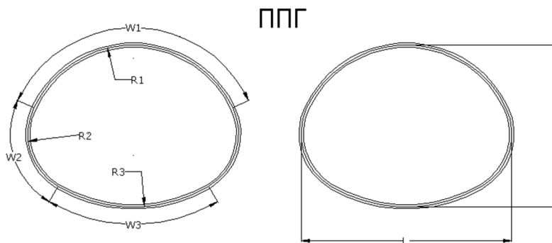
Рисунок 1.2 - ППГ - Полицентрические Пониженные Горизонтальные
