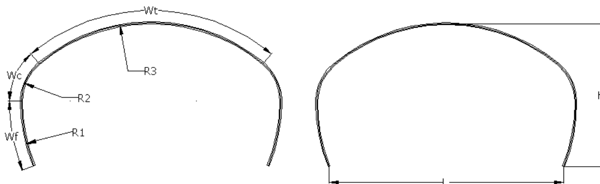
Рисунок 5.85 - Арочные полицентрические высокие, профиль 150x50
