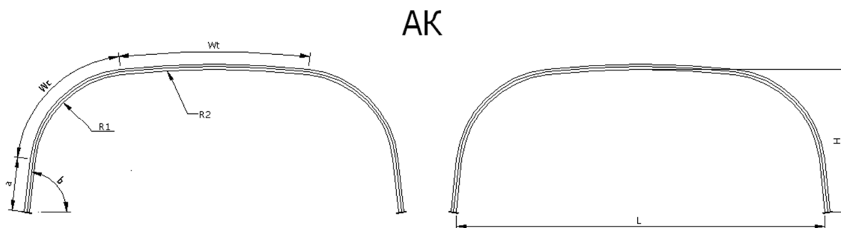
Рисунок 1.11 – АК – Арочные Коробчатые
