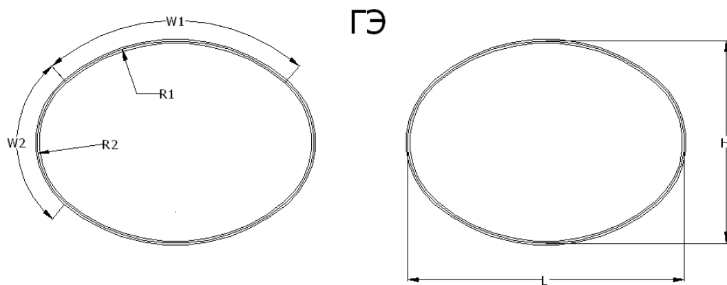
Рисунок 5.8 - Горизонтальные эллиптические, профиль 150x50
