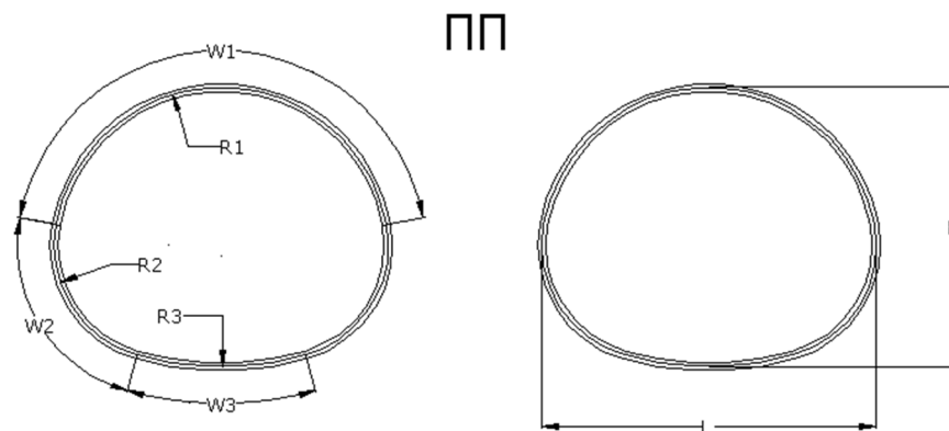
Рисунок 1.1 - ПП - Полицентрические Пониженные
