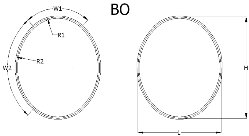
Рисунок 5.7 - Вертикальные овальные, профиль 150x50
