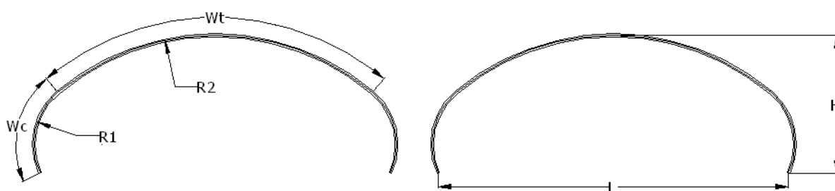
Рисунок 5.14 - Арочные полицентрические средние, профиль 150x50
