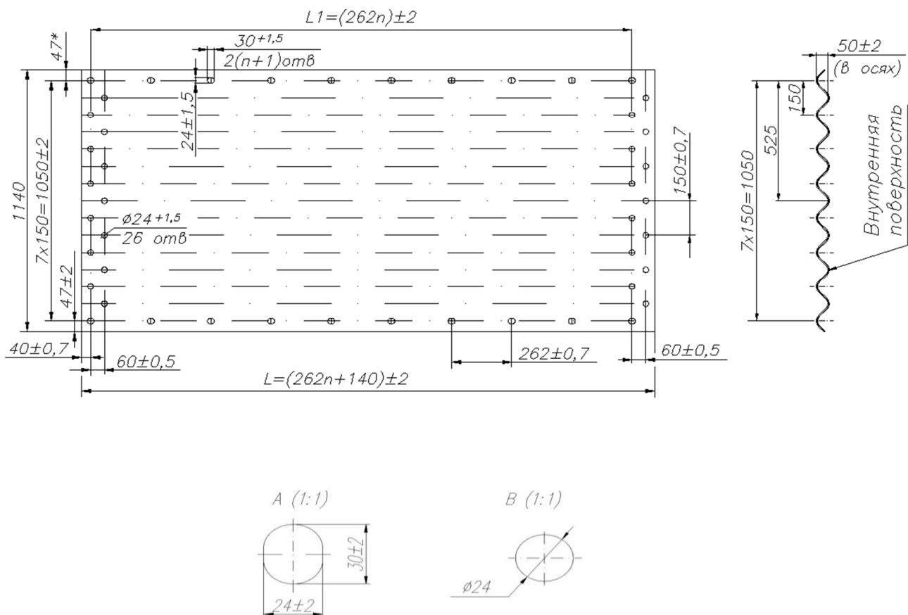
Рисунок 4.2 - Листы гофрированные
