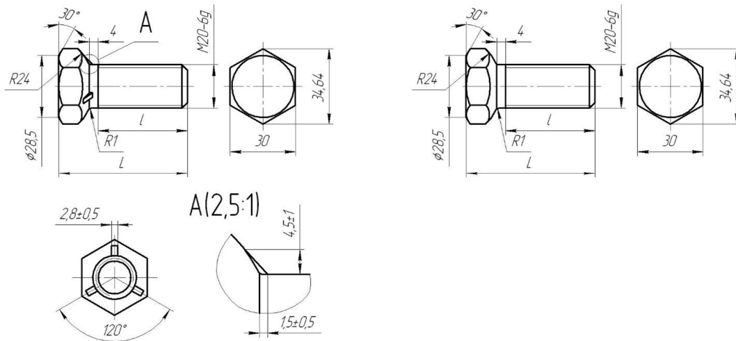
Рисунок 5.1 - Соединительные болты
