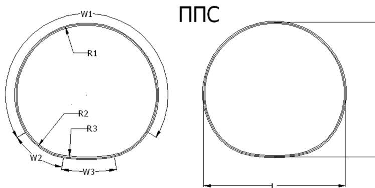
Рисунок 1.4 - ППС - Полицентрические Повышенные Средние
