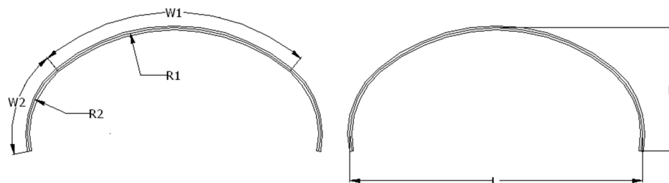
Рисунок 1.13 – АПН – Арочные Полицентрические Низкие
