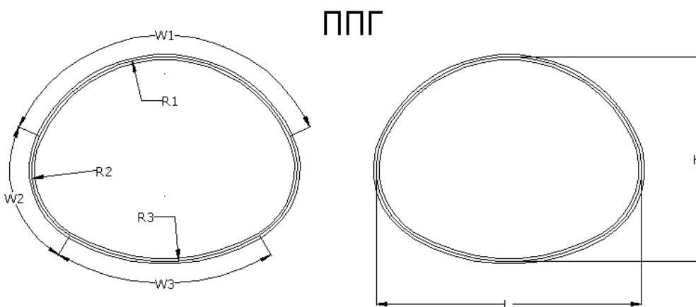
Рисунок 5.2 -Полицентрические пониженные горизонтальные, профиль 150x50
