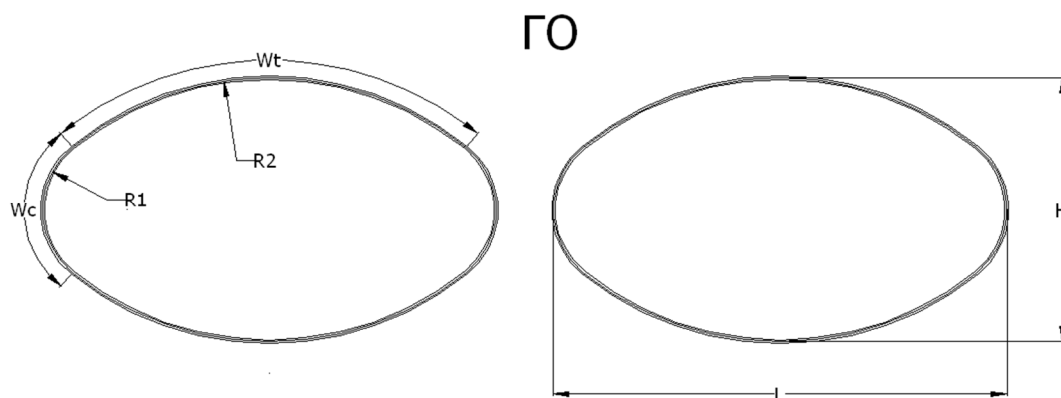
Рисунок 1.9 – ГО – Горизонтальные Овальные
