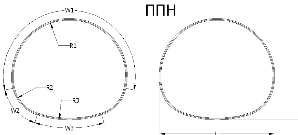
Рисунок 5.3 -Полицентрические повышенные низкие, профиль 150x50
