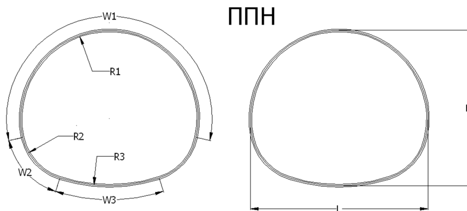
Рисунок 1.3 - ППН - Полицентрические Повышенные Низкие
