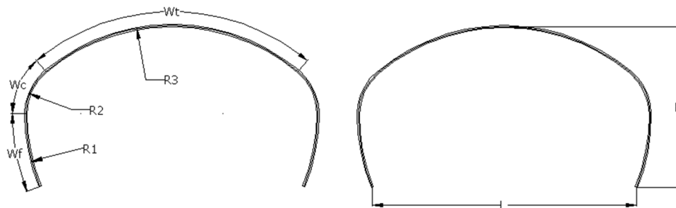
Рисунок 1.15 – АПВ – Арочные Полицентрические Высокие
