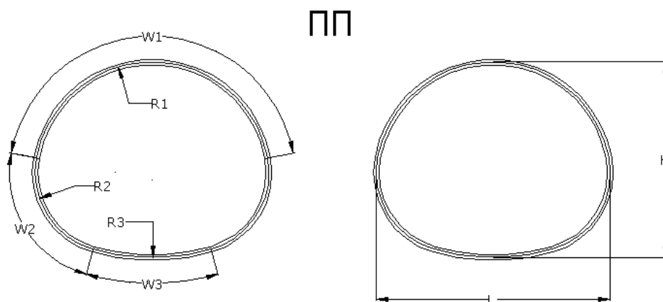
Рисунок 5.1 Полицентрические пониженные, профиль 150x50
