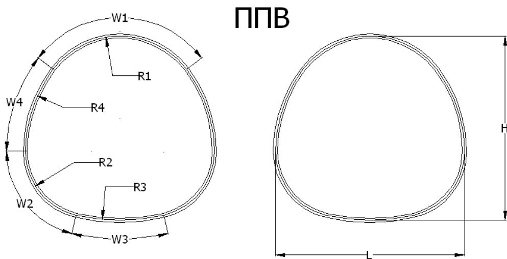
Рисунок 5.5 - Полицентрические повышенные высокие, профиль 150x50
