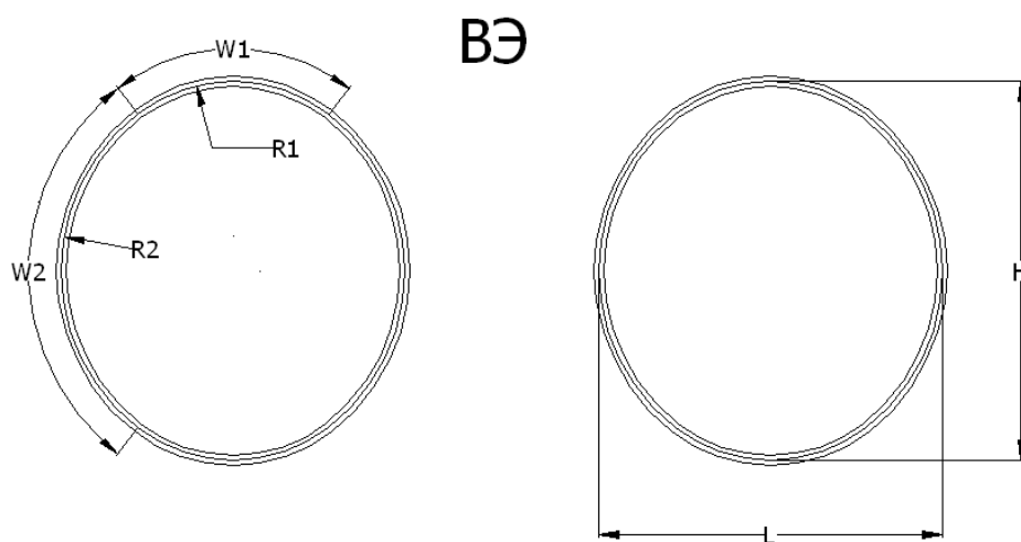
Рисунок 5.6 - Вертикальные эллиптические, профиль 150x50
