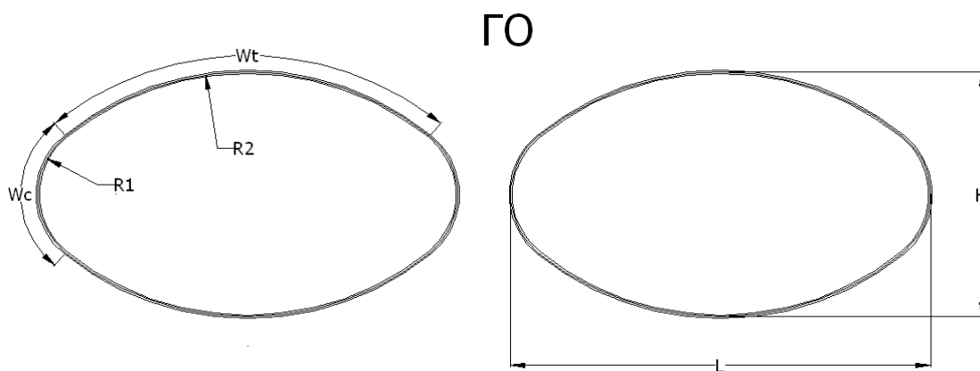
Рисунок 5.9 - Горизонтальные овальные, профиль 150x50
