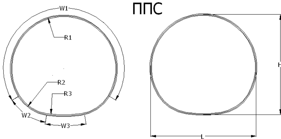
Рисунок 5.4 - Полицентрические повышенные средние, профиль 150x50
