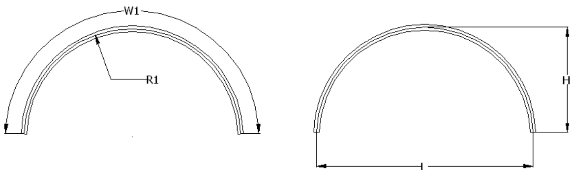
Рисунок 5.12 Арочные радиусные, профиль 150x50
