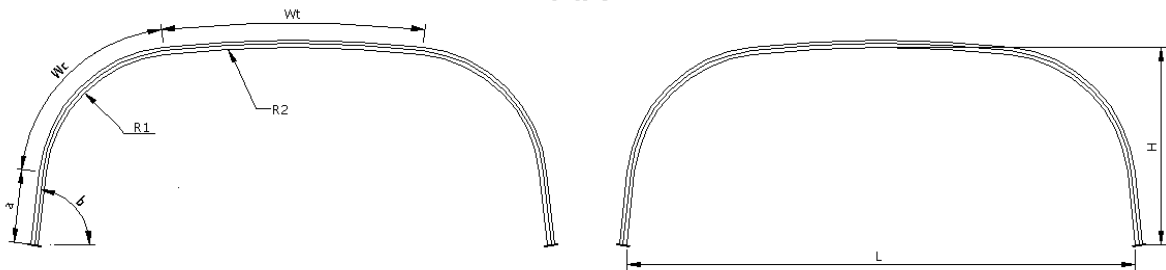
Рисунок 5.11 - Арочные коробчатые, профиль 150x50
