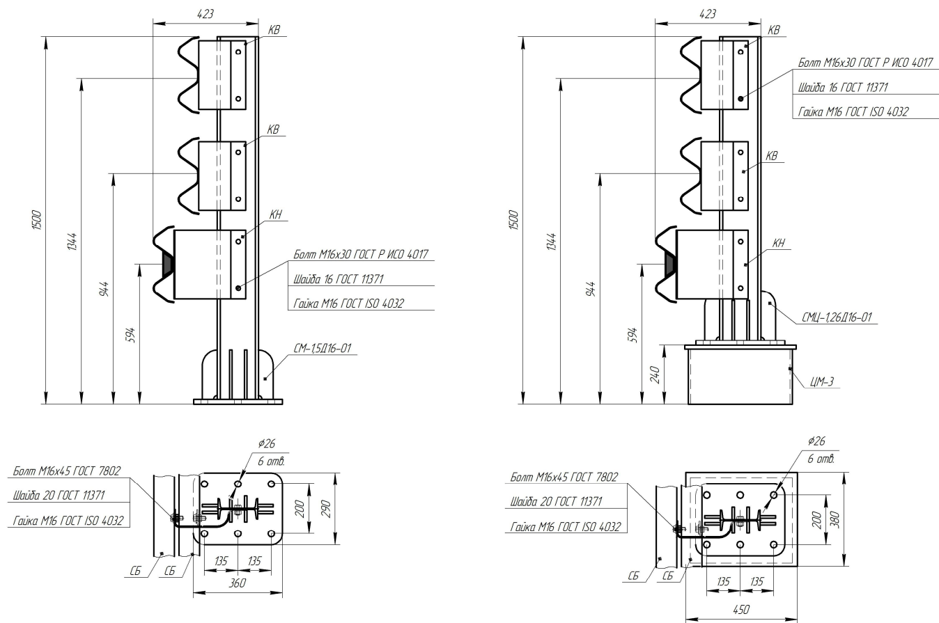
Рисунок В.92 –Мостовое ограждение 21МО/500÷600-1,5xS(Д16); 21МО/500÷600-1,5(Ц)xS(Д16)
