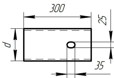
Рисунок Г.12 - Вставка стыковая (ВС)
