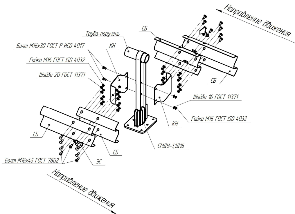
Рисунок В.110 – Схема сборки мостового ограждения 21МД/350÷450-1,1(У)хS(Д16)
