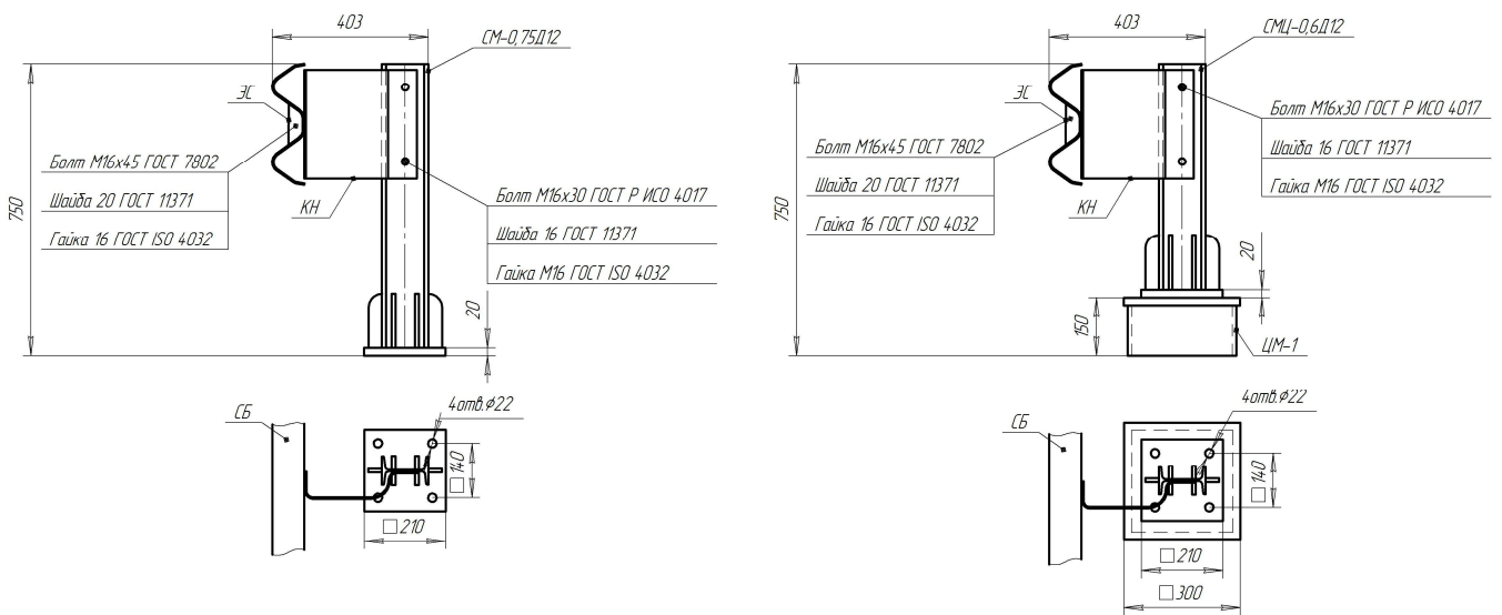
Рисунок В.14 - Мостовое ограждение 21МО/130÷300-0,75xS(Д12); 21МО/130÷300-0,75(Ц)xS(Д12)
