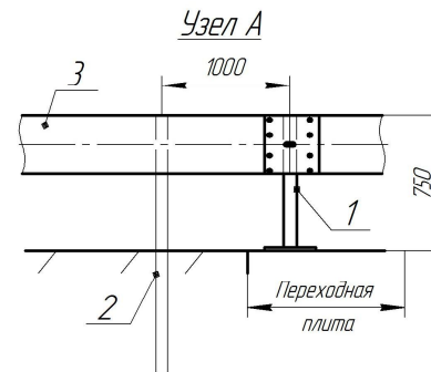
Рисунок В.113 - Сопряжение дорожной группы 11ДО(У1-У4) с мостовой группой 11МО(У1-У3)
