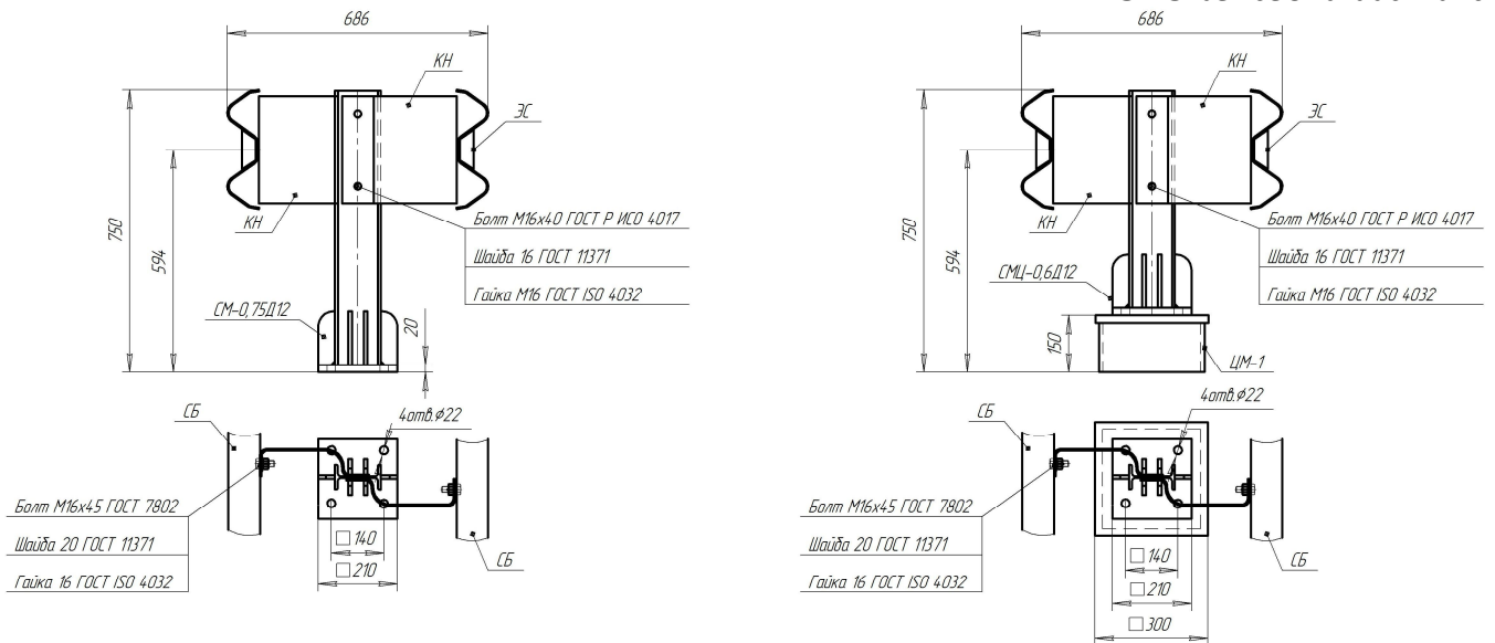
Рисунок В.20 - Мостовое ограждение 21МД/130÷300-0,75xS(D12); 21МД/130÷300-0,75(Ц)xS(D12)
