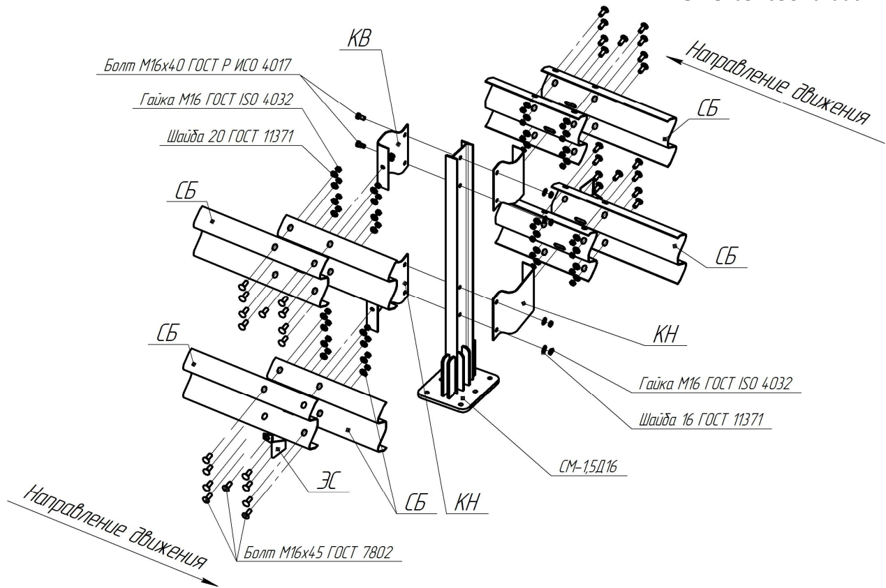
Рисунок В.87 – Схема сборки мостового ограждения 21МД/500÷550-1,5
