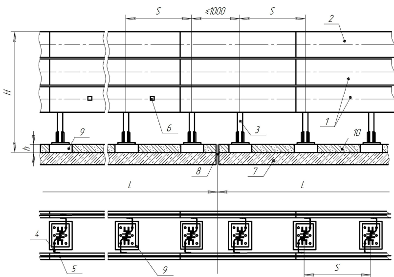
Рисунок В.12 - Ограждение группы 21МД/500-600(Ц)
