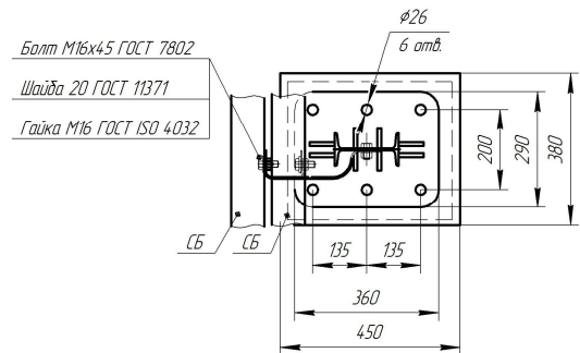
Рисунок В.83 - Мостовое ограждение 21МО/500÷600-1,5xS(D16); 21МО/500÷600-1,5(Ц)xS(D16)
