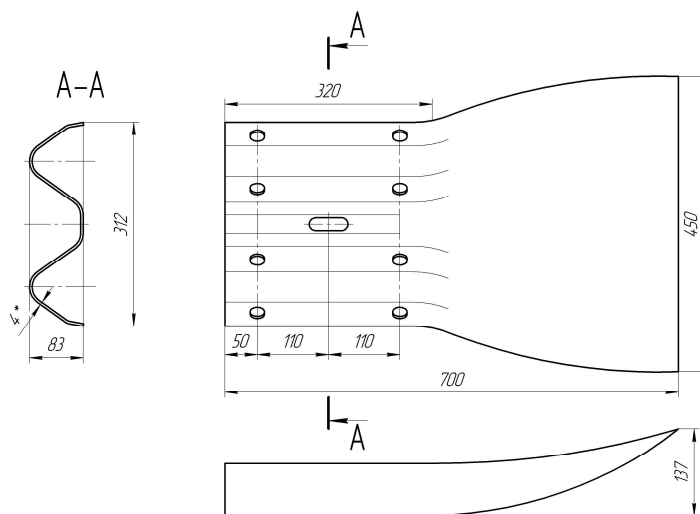
Рисунок Г.8 – Элемент концевой (ЭК-1)
