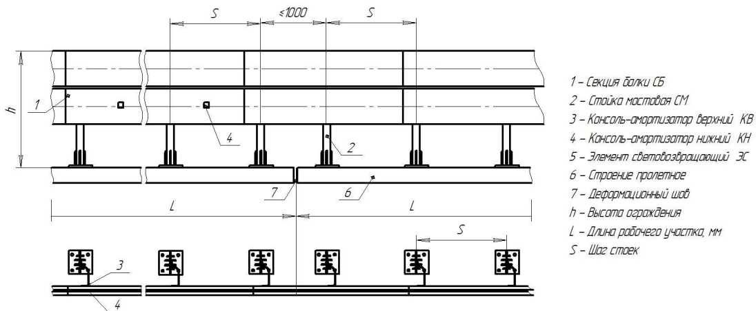
Рисунок В.3 - Ограждение группы 21МО/300-600
