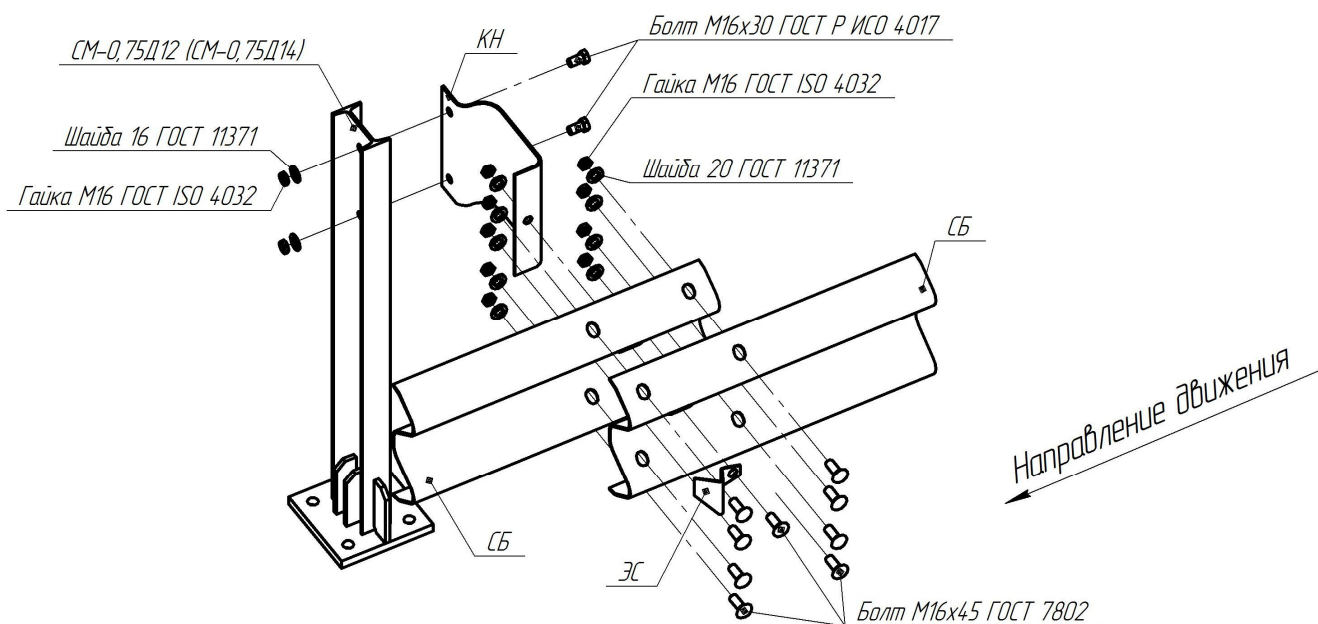
Рисунок В.15 – Схема сборки мостового ограждения 21МО/130÷300-0,75
