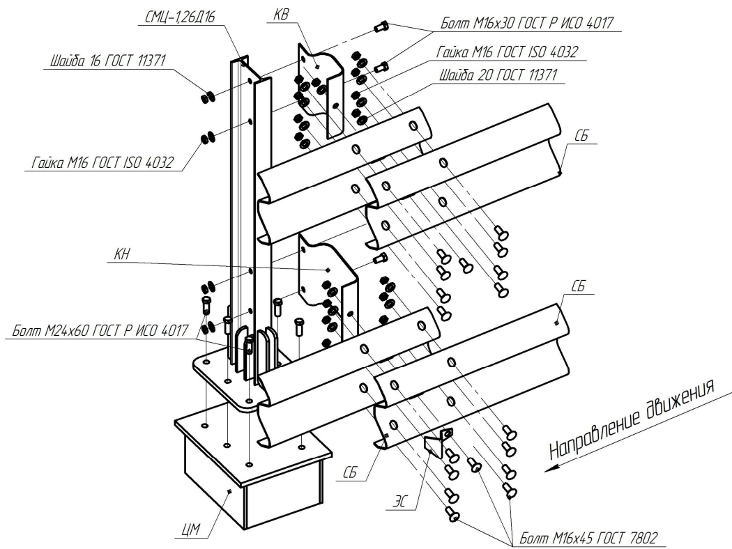
Рисунок В.85 – Схема сборки мостового ограждения 21МО/500÷600-1,5(Ц)
