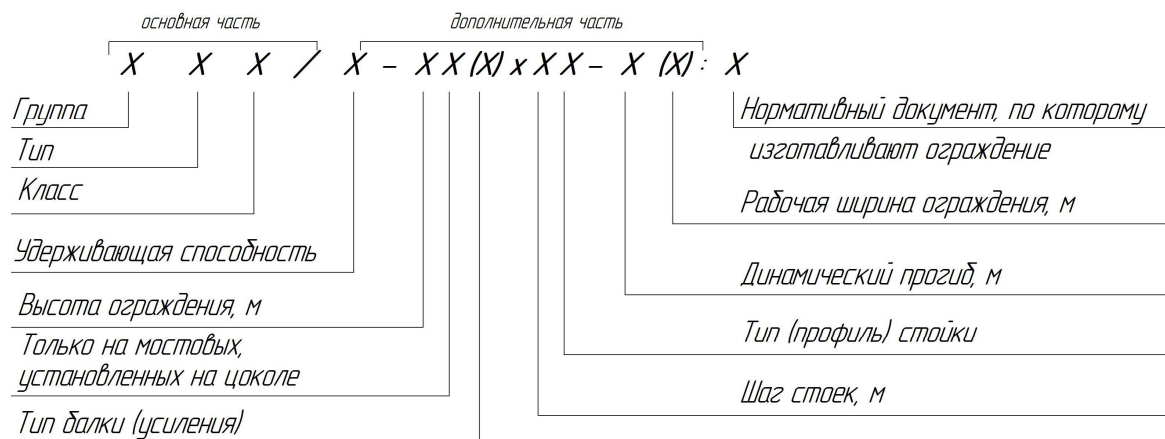
Рисунок 5.1- Маркировка ограждений
