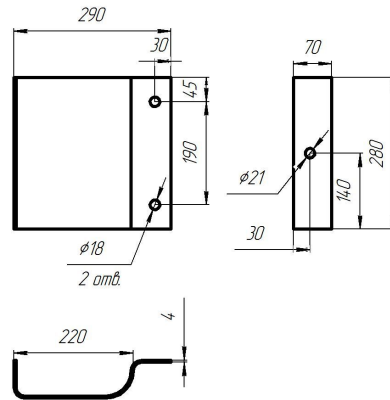
Рисунок Г.1 – Консоль-амортизатор нижний (КН)
