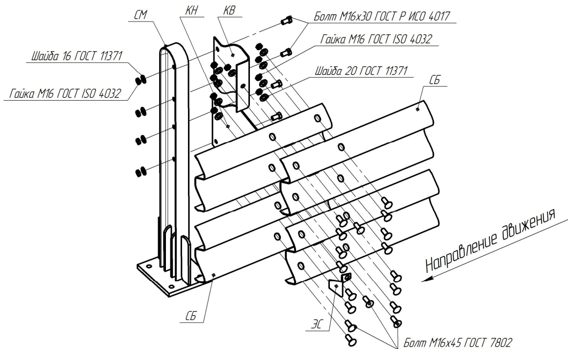
Рисунок В.42 – Схема сборки мостового ограждения 21МО/300÷450-1,1
