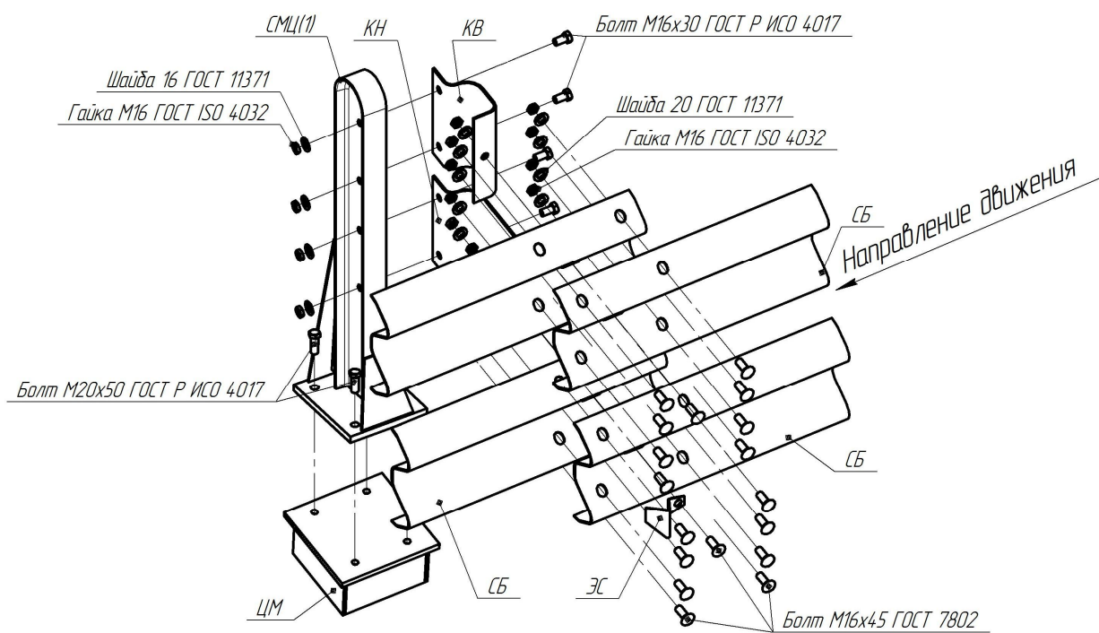
Рисунок В.59 – Схема сборки мостового ограждения 21МО/300÷450-0,9÷1,1(Ц)
