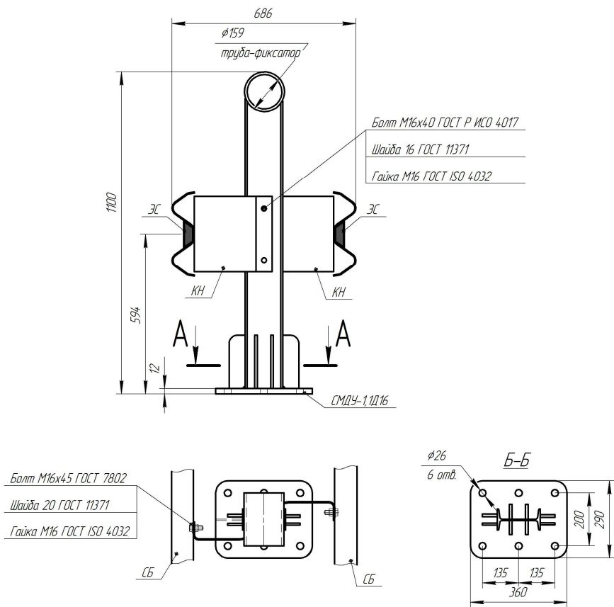
Рисунок В.109 – Мостовое ограждение 21МД/350÷450-1,1(У)хS(Д16)
