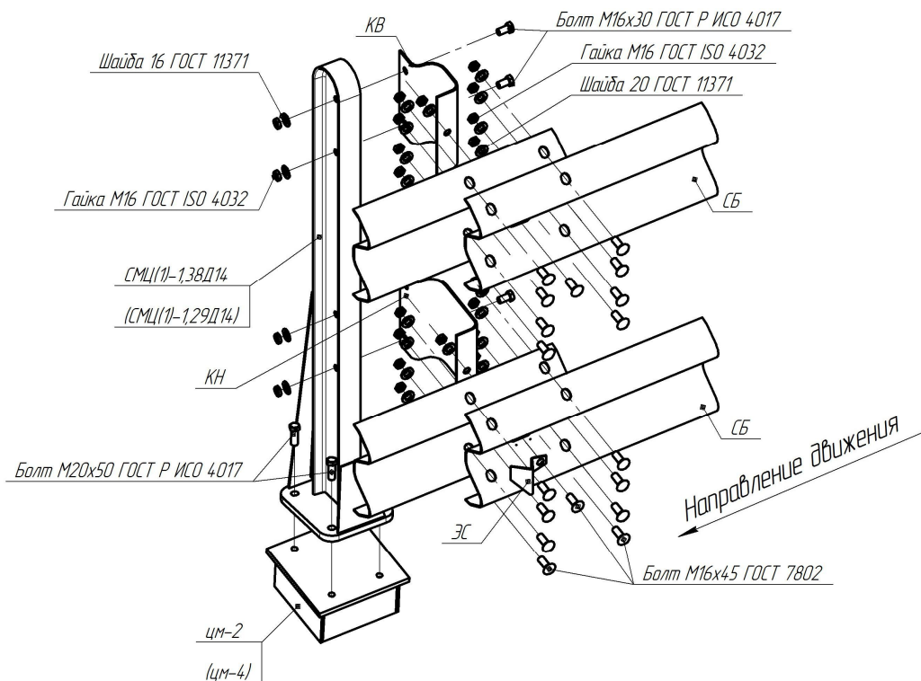
Рисунок В.82 – Схема сборки мостового ограждения 21МО/450÷500-1,5(Ц)
