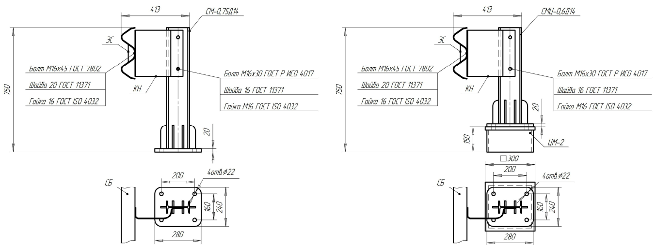
Рисунок В.13 - Мостовое ограждение 21МО/130÷300-0,75xS(Д14); 21МО/130÷300-0,75(Ц)xS(Д14)
