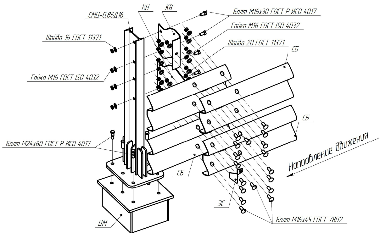
Рисунок В.72 – Схема сборки ограждения мостового 21МО/500÷600-1,1(Ц)
