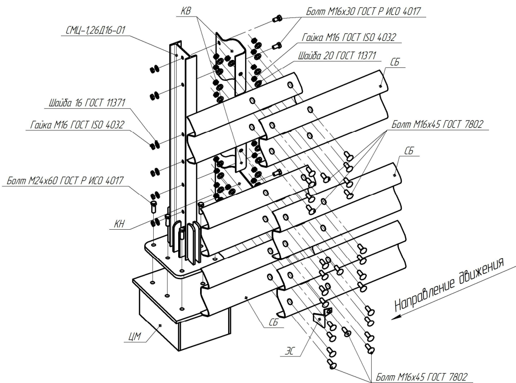
Рисунок В.93 –Схема сборки мостового ограждения 21МО/500÷600-1,5xS(Д16)
