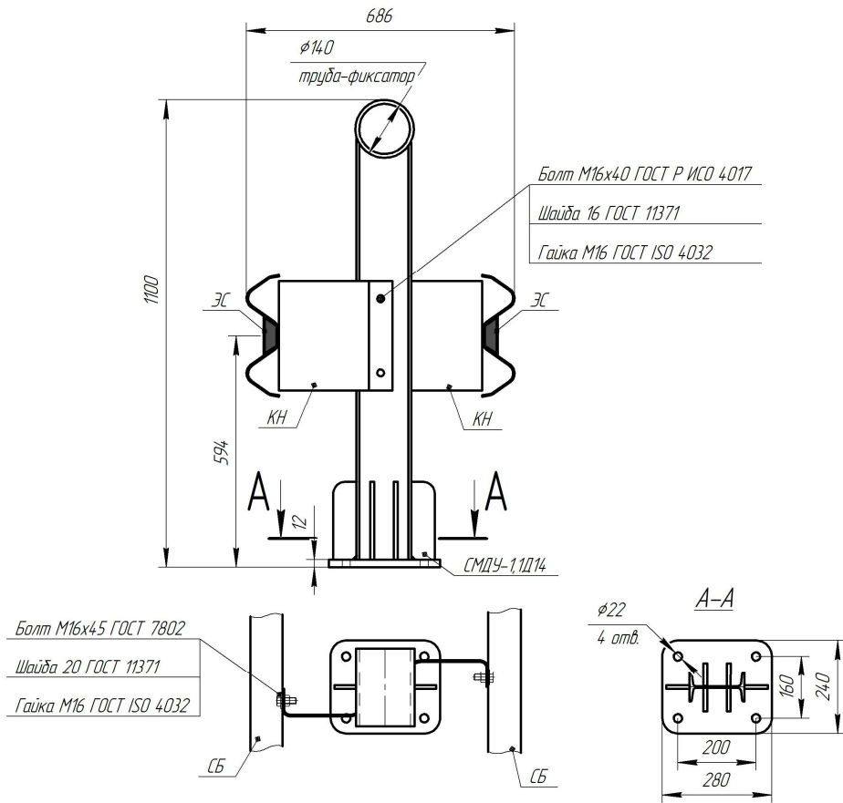
Рисунок В.107 –Мостовое ограждение 21МД/350÷450-1,1(У)хS(Д14)
