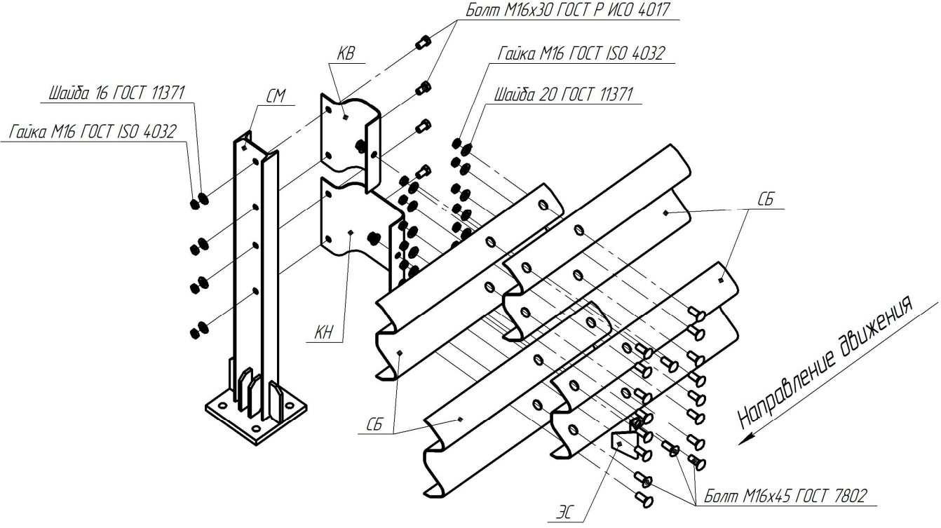
Рисунок В.32 – Схема сборки мостового ограждения 21МО/300÷450-1,1
