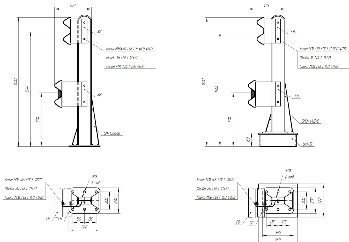
Рисунок В.89 – Мостовое ограждение 21МО/600-1,5х2,0Д16-0,59(0,88) 21МО/600-1,5(Ц)х2,0Д16-0,59(0,68)
