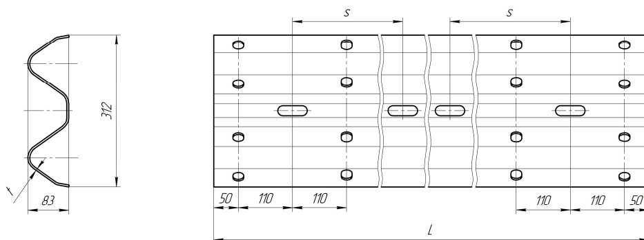
Рисунок Г.2 – Консоль-амортизатор верхний (КВ)
