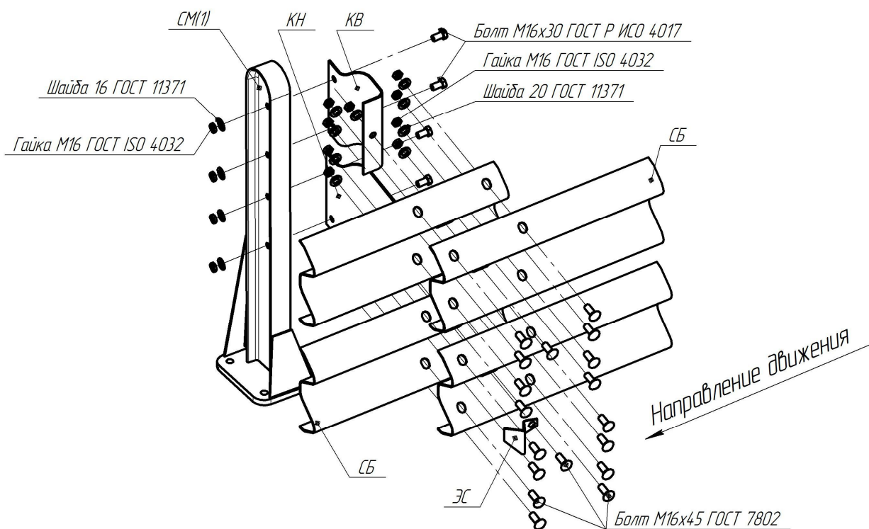
Рисунок В.58 – Схема сборки мостового ограждения 21МО/300÷450-0,9÷1,1
