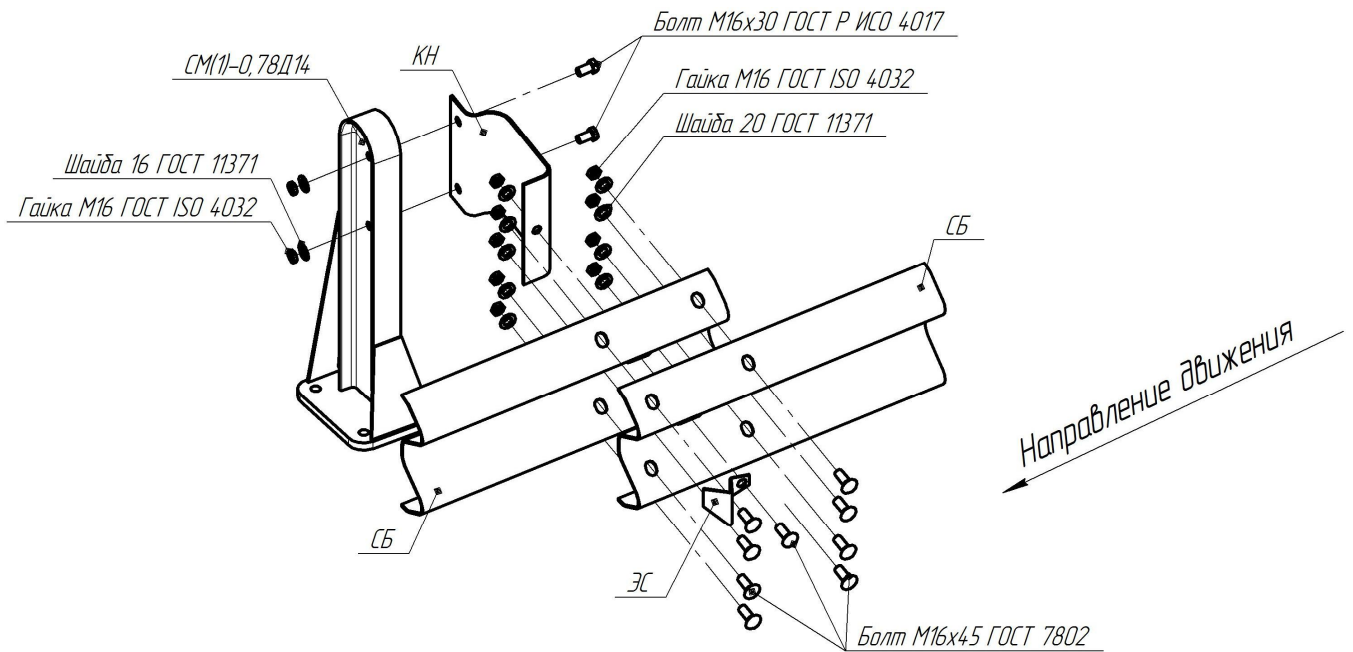
Рисунок В.18 – Схема сборки мостового ограждения 21МО/130÷300-0,75
