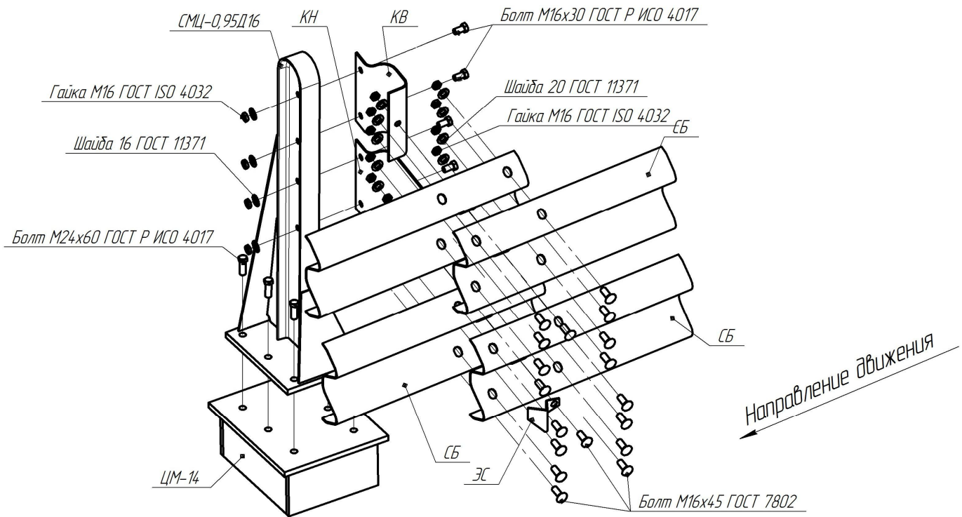
Рисунок В.79 – Схема сборки мостового ограждения 21МО/500÷600-1,1(Ц)
