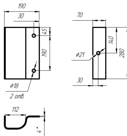
Рисунок Г.2 – Консоль-амортизатор верхний (КВ)
