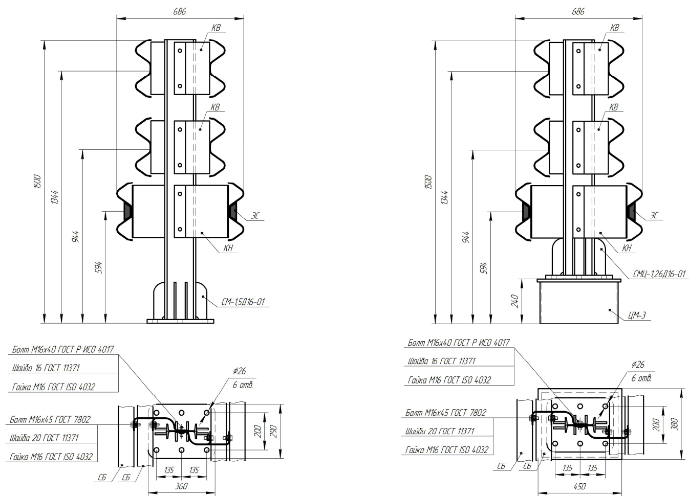
Рисунок В.95 – Мостовое ограждение 21МД/500÷600-1,5xS(Д16); 21МО/500÷600-1,5(Ц)xS(Д16)
