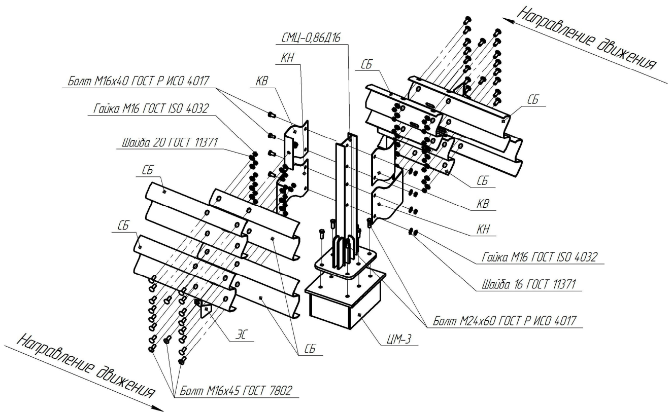
Рисунок В.75 – Схема сборки мостового ограждения 21МД/500÷550-1,1(Ц)
