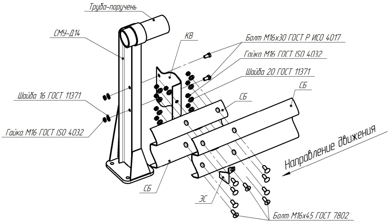
Рисунок В.100 –Схема сборки мостового ограждения 21МО/350÷450-0,95÷1,1(У)хS(Д14)
