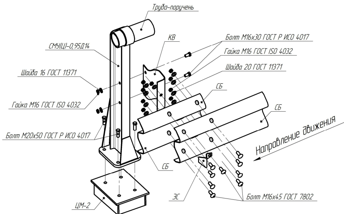
Рисунок В.104 –Схема сборки мостового ограждения 21МО/350÷450-1,1(УЦ)хS(Д14)
