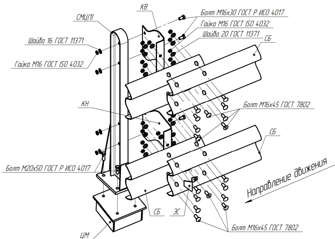
Рисунок В.66 – Схема сборки мостового ограждения 21МО/500-1,3(Ц)
