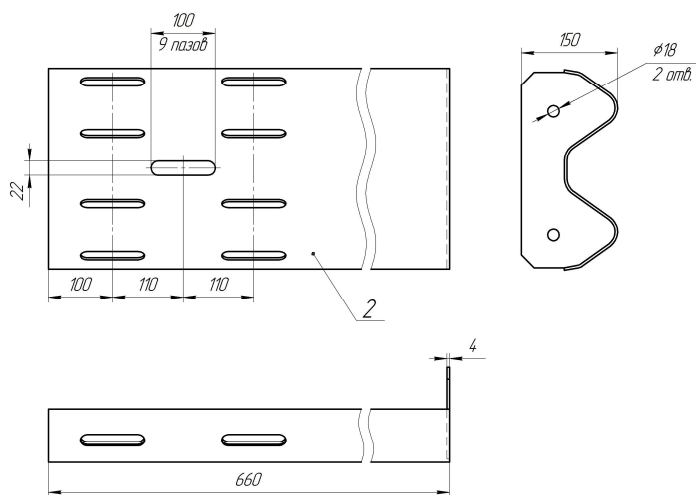
Рисунок Г.9 – Элемент концевой (ЭК-3)
