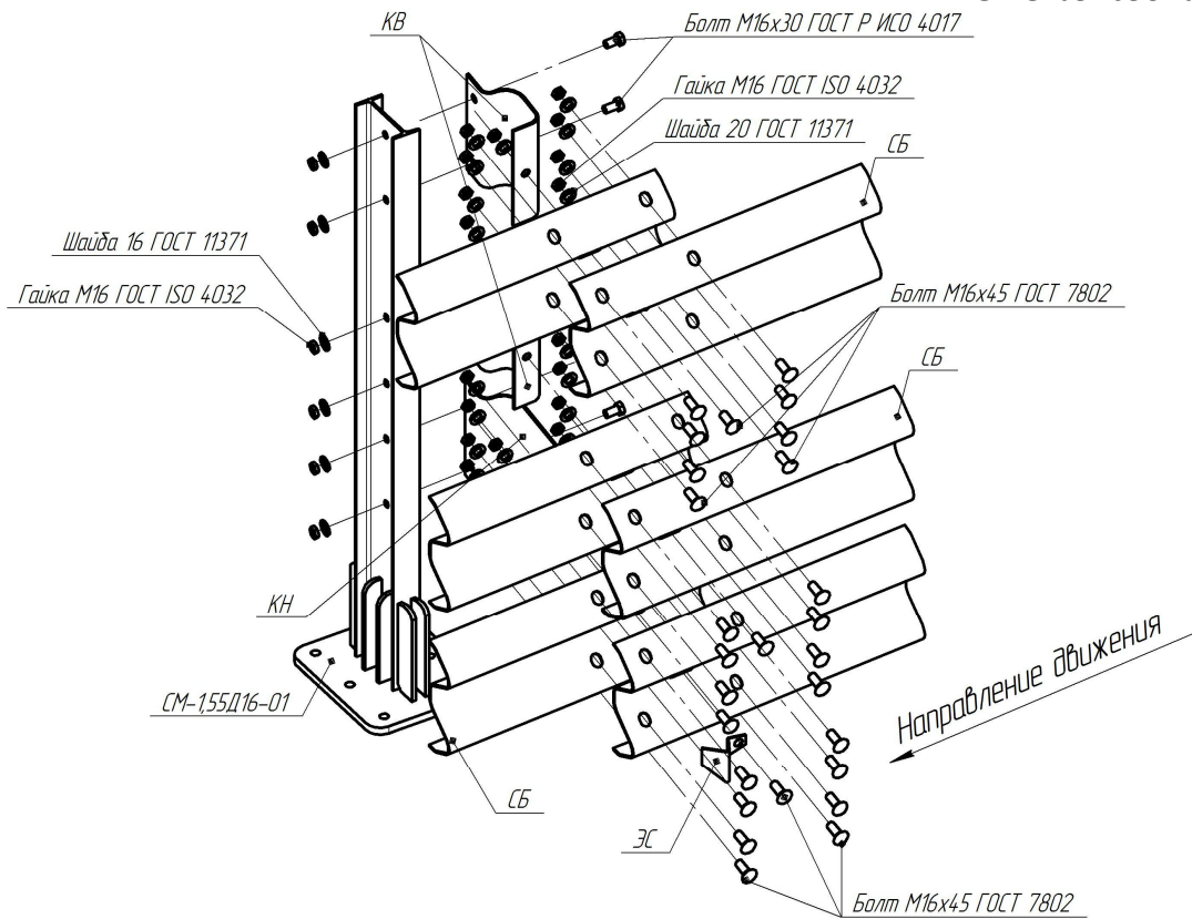
Рисунок В.93 –Схема сборки мостового ограждения 21МО/500÷600-1,5xS(Д16)
