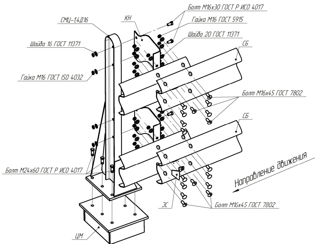
Рисунок В.91 – Схема сборки мостового ограждения 21МО/600-1,5(Ц)х2,0Д16-0,59(0,68)
