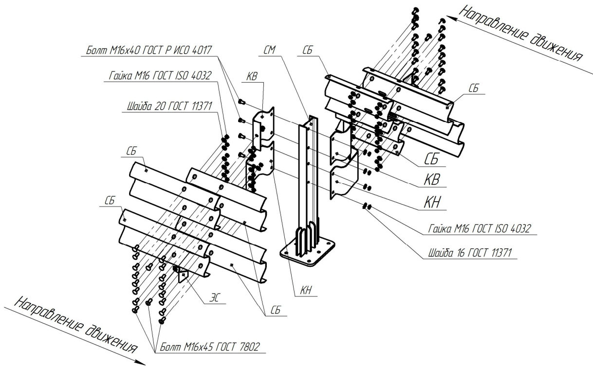
Рисунок В.74 – Схема сборки мостового ограждения 21МД/500÷550-1,1
