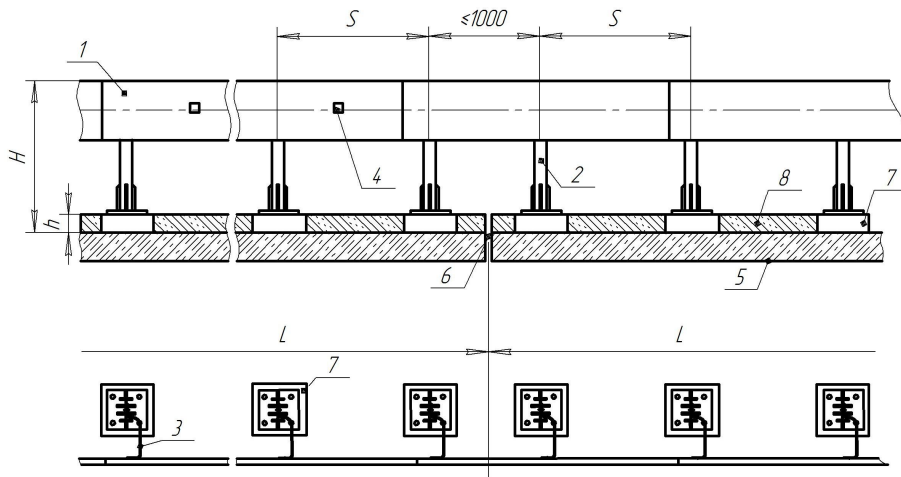
Рисунок В.7 - Ограждение группы 21МО/130-300(Ц)
