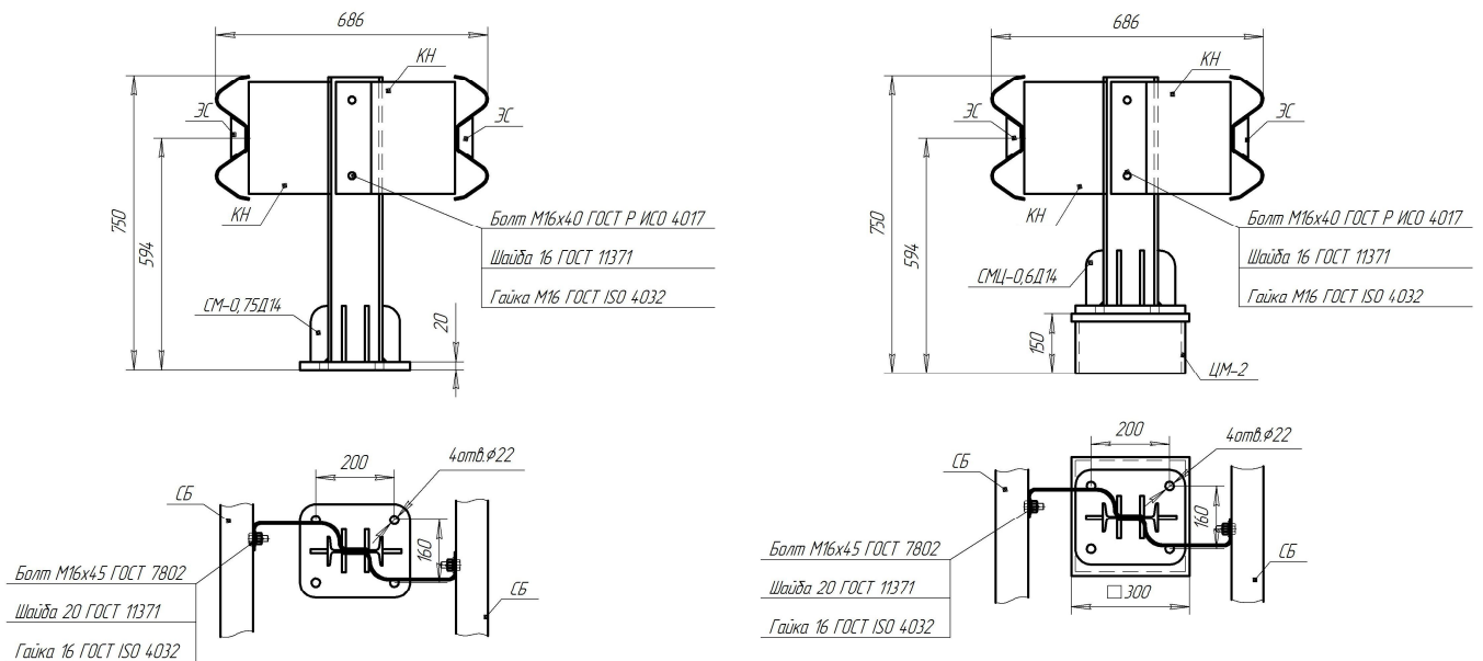
Рисунок В.21 - Мостовое ограждение на цоколе 21МД/130÷300-0,75xS(D14); 21МД/130÷300-0,75(Ц)xS(D14)
