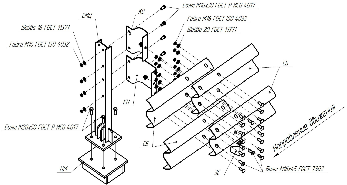
Рисунок В.36 – Схема сборки мостового ограждения на цоколе 21МО/300÷450(Ц)
