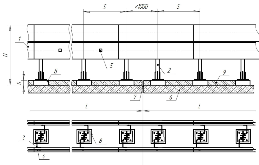
Рисунок В.10 - Ограждение группы 21МД/300-600(Ц)
