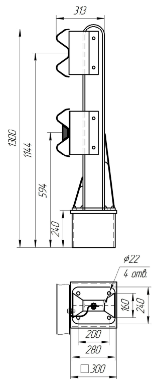
Рисунок 5.71 (СМЦ(1)-1,09Д14) без КН ЦМ-4
