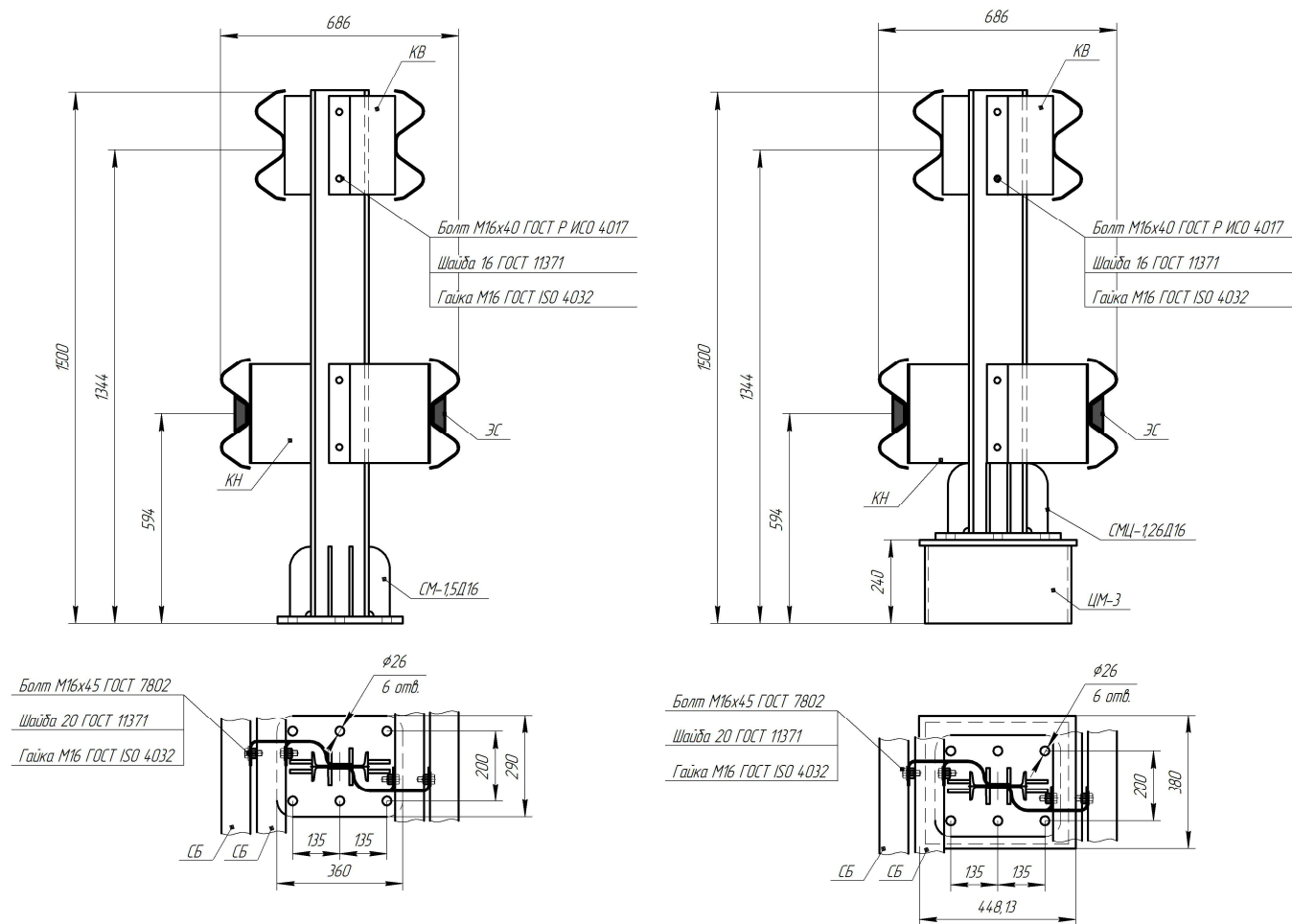
Рисунок В.86 - Мостовое ограждение 21МД/500÷550-1,5xS(Д16); 21МД/500÷550-1,5(Ц)xS(Д16)
