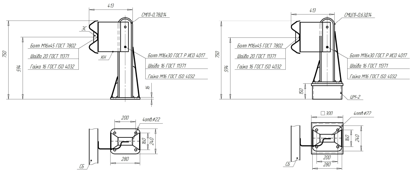
Рисунок В.17 - Мостовое ограждение 21МО/130÷300-0,75xS(Д14); 21МО/130÷300-0,75(Ц)xS(Д14)
