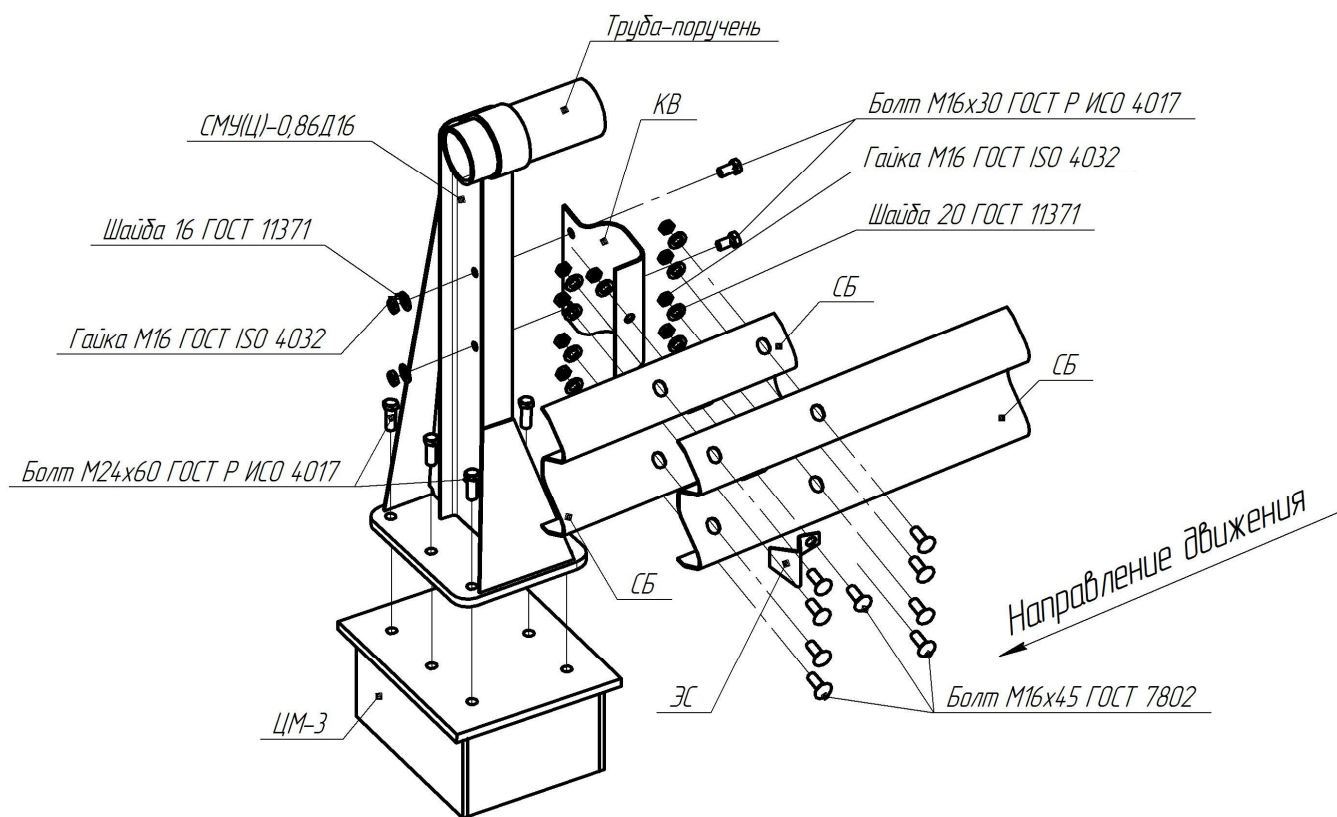
Рисунок В.106 – Схема сборки мостового ограждения 21МО/350÷450-1,1(УЦ)хS(Д16)
