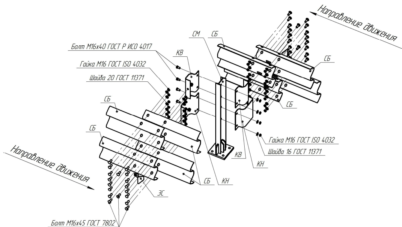
Рисунок В.39 – Схема сборки мостового ограждения 21МД/300÷450-1,1(Д14)
