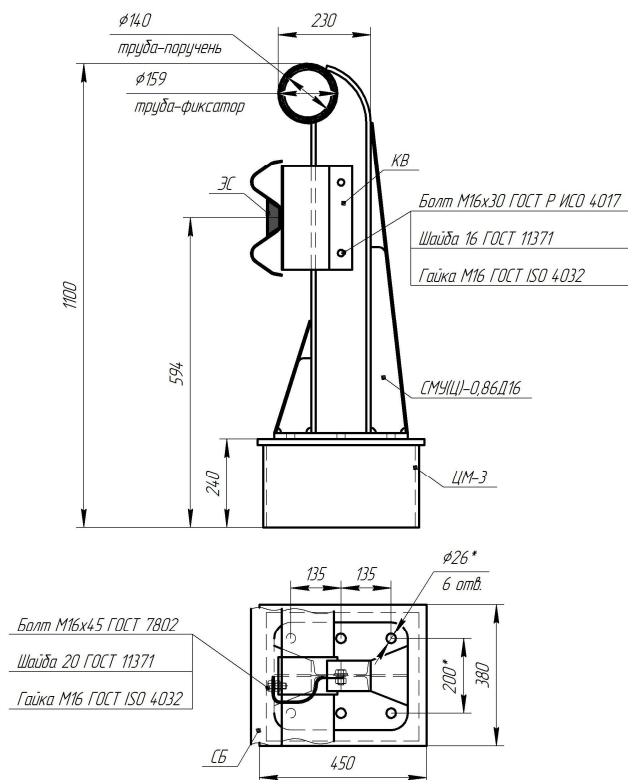
Рисунок В.105 – Мостовое ограждение 21МО/350÷450-1,1(УЦ)хS(Д16)
