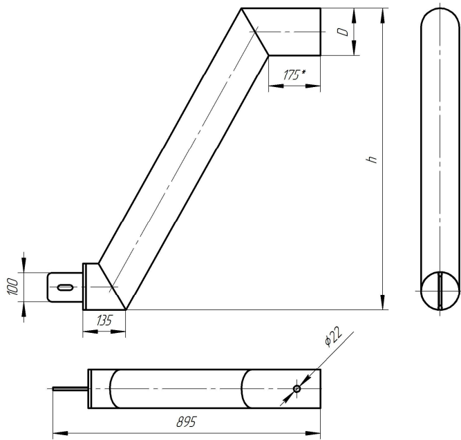
Рисунок Г.13 - Поручень концевой ПК-2
