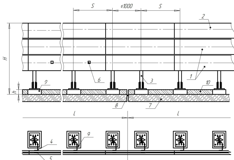
Рисунок В.11 - Ограждение группы 21МО/500-600(Ц)
