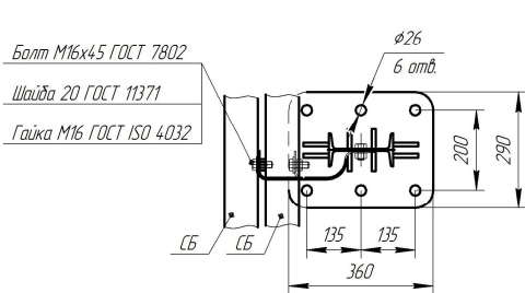
Рисунок В.83 - Мостовое ограждение 21МО/500÷600-1,5xS(D16); 21МО/500÷600-1,5(Ц)xS(D16)
