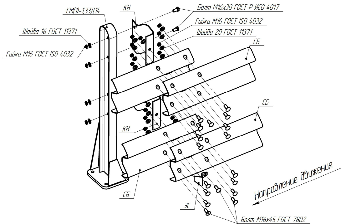
Рисунок В.65 – Схема сборки мостового ограждения 21МО/500-1,3
