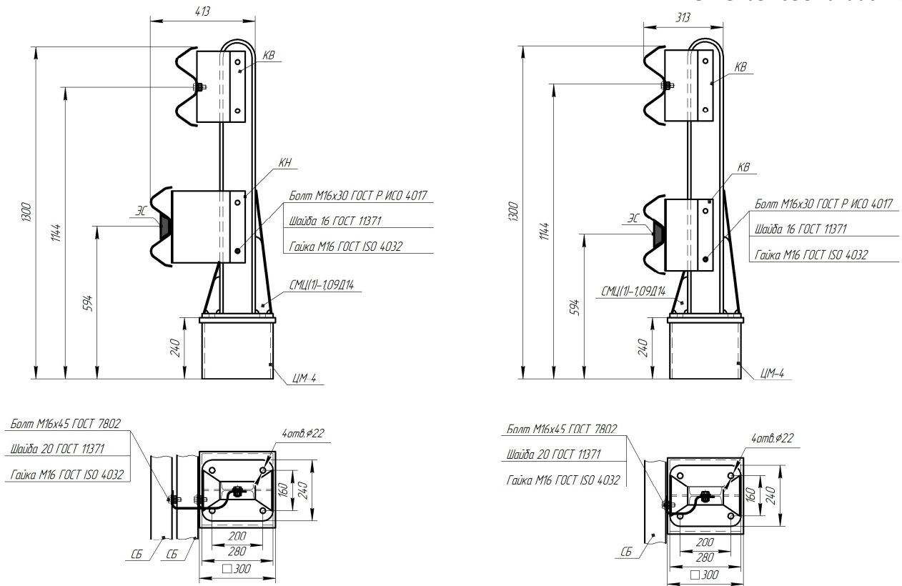
Рисунок В.64- Мостовое ограждение 21МО/500-1,3(Ц)x1,0Д14-0,46(0,85); 21МО/500-1,3(Ц)x1,0Д14-0,46(0,88)
