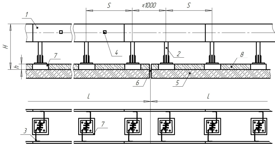
Рисунок В.8 - Ограждение группы 21МД/130-300(Ц)
