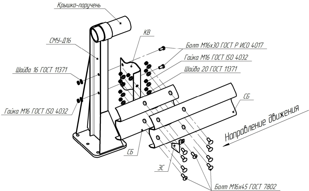
Рисунок В.102 – Схема сборки мостового ограждения 21МО/350÷450-0,95÷1,1(У)хS(Д16)
