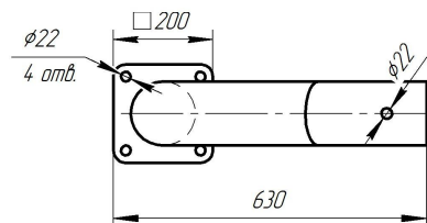
Рисунок Г.14 – Труба усиления концевая (ТК-2)
