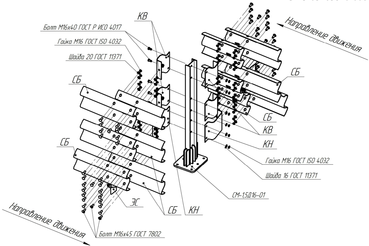
Рисунок В.96 –Схема сборки мостового ограждения 21МД/500÷600-1,5
