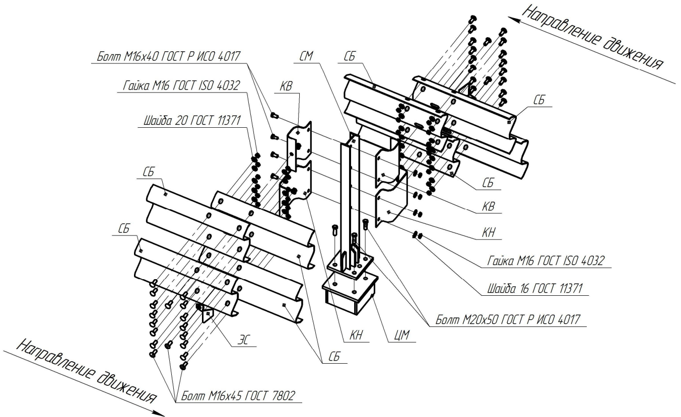
Рисунок В.40 – Схема сборки мостового ограждения 21МД/300÷450-1,1(Ц)
