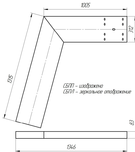
Рисунок Г.5 – Секция балки переходная правая (левая) СБПП (СБПЛ)
