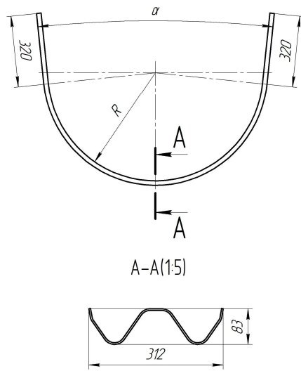
Рисунок Г.6 – Секция балки радиусная выпуклая (СБР-1)
