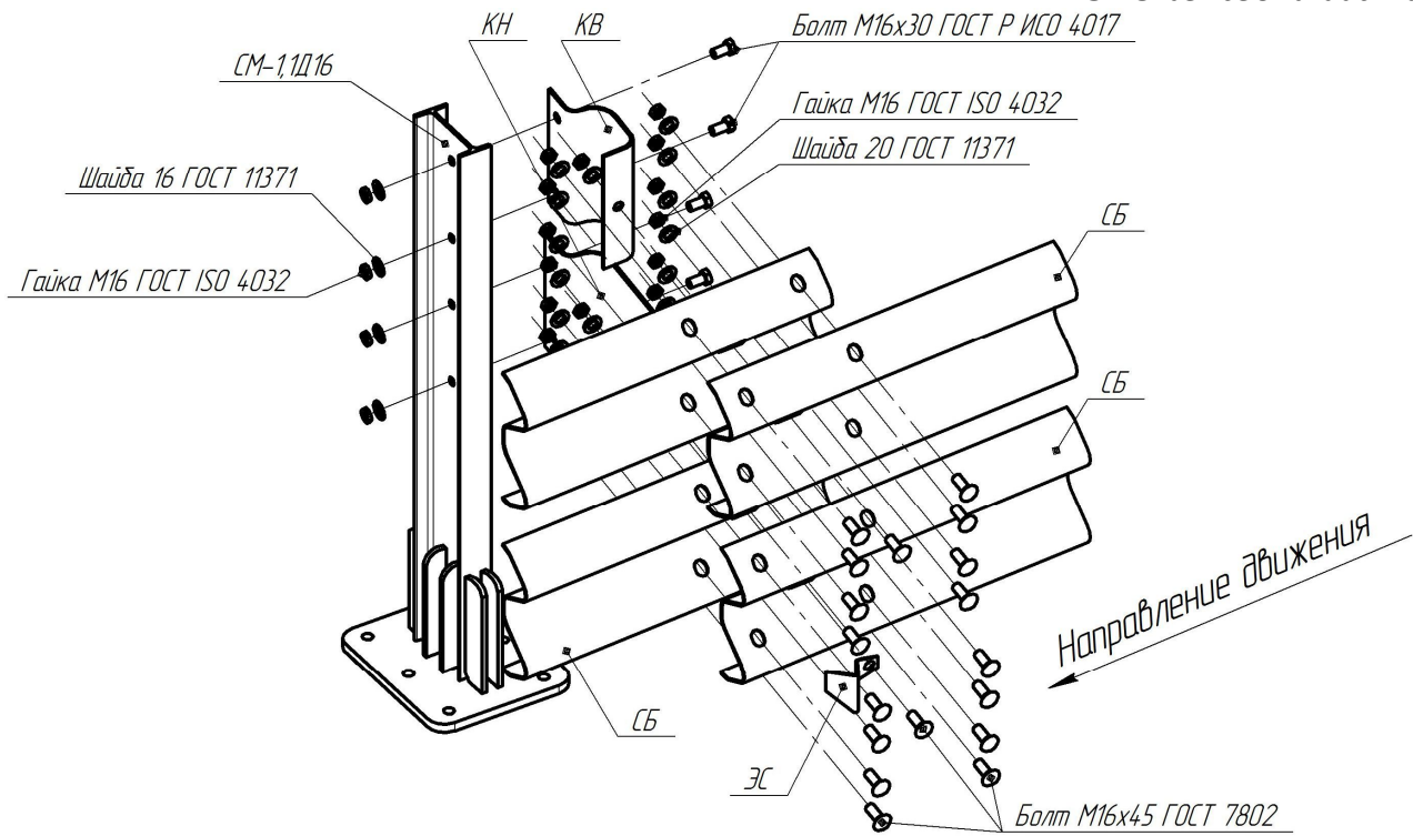
Рисунок В.71 – Схема сборки ограждения мостового 21МО/500÷600-1,1
