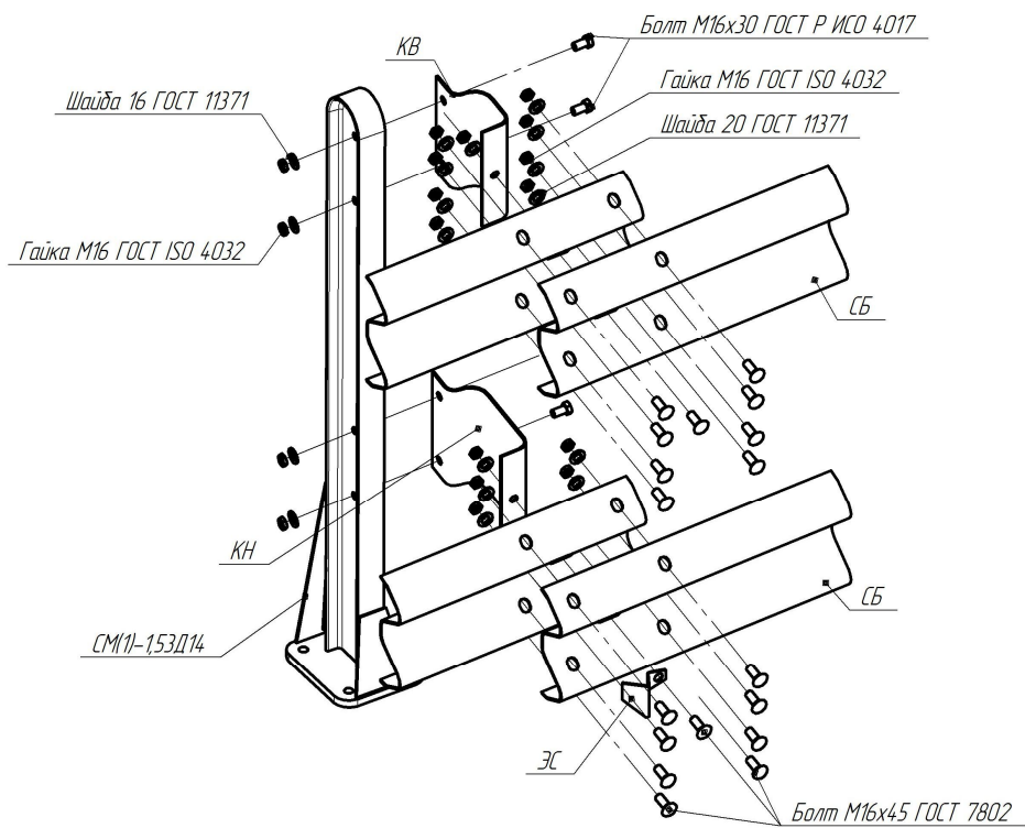
Рисунок В.81 – Схема сборки мостового ограждения 21МО/450÷500-1,5
