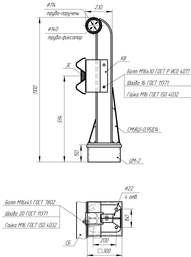
Рисунок В.103 –Мостовое ограждение 21МО/350÷450-1,1(УЦ)хS(Д14)
