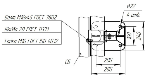
Рисунок В.98 –Мостовое ограждение 21МО/350÷400-0,95(У)хS(Д14)
