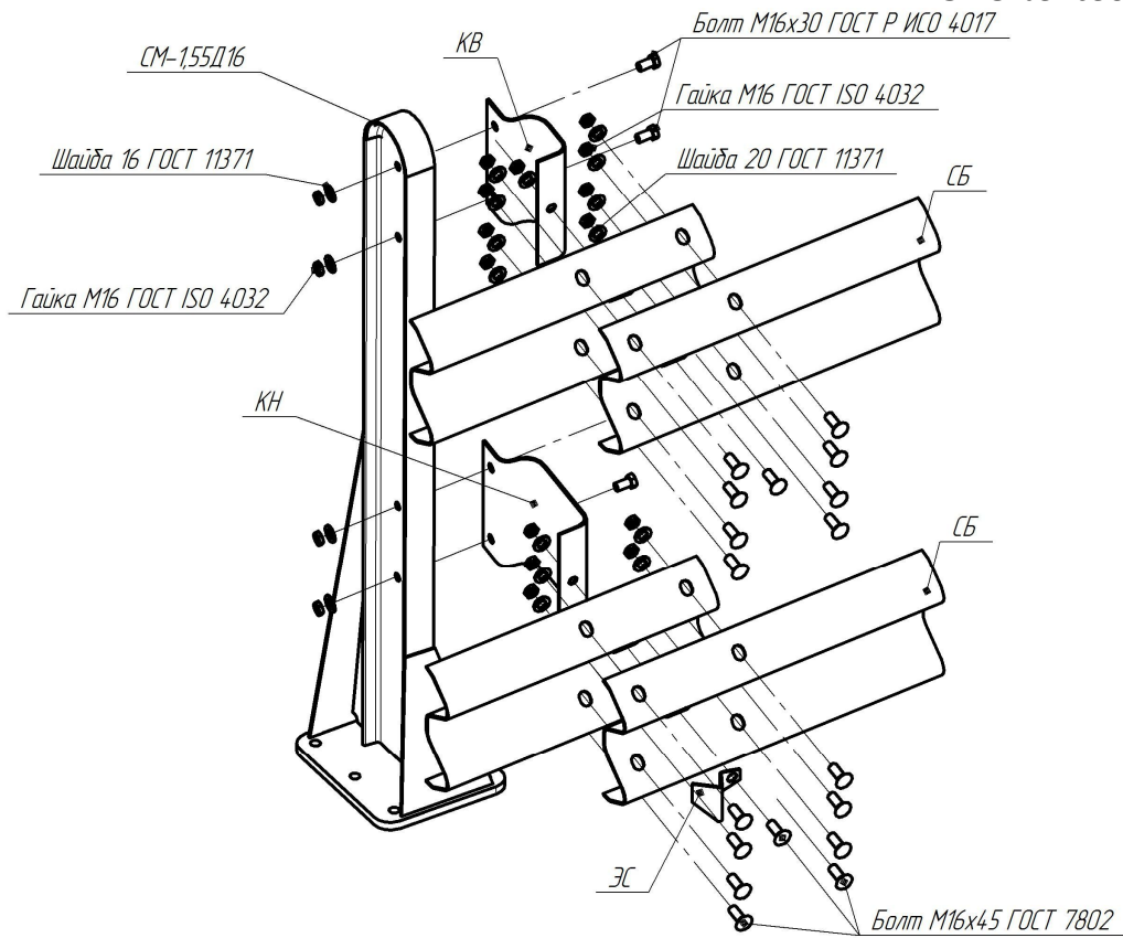
Рисунок В.90 – Схема сборки мостового ограждения 21МО/600-1,5х2,0Д16-0,59(0,88)
