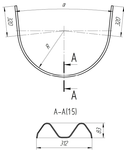
Рисунок Г.7 – Секция балки радиусная вогнутая (СБР-2)
