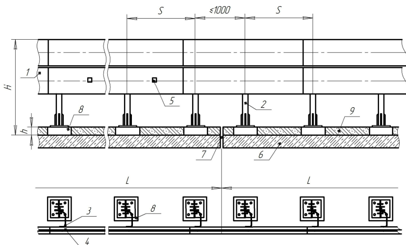
Рисунок В.9 - Ограждение группы 21МО/300-600(Ц)
