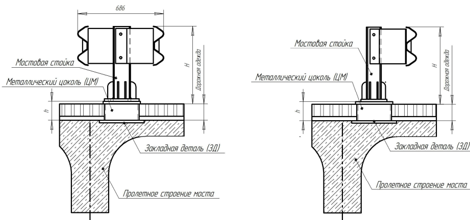
Рисунок Б.1 – Схема установки двустороннего и одностороннего
