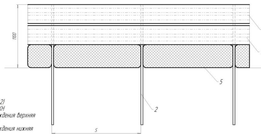
Ограждение с нижней металлической сеткой
