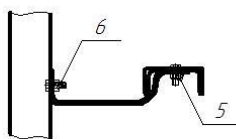
Стойка из двутавра
