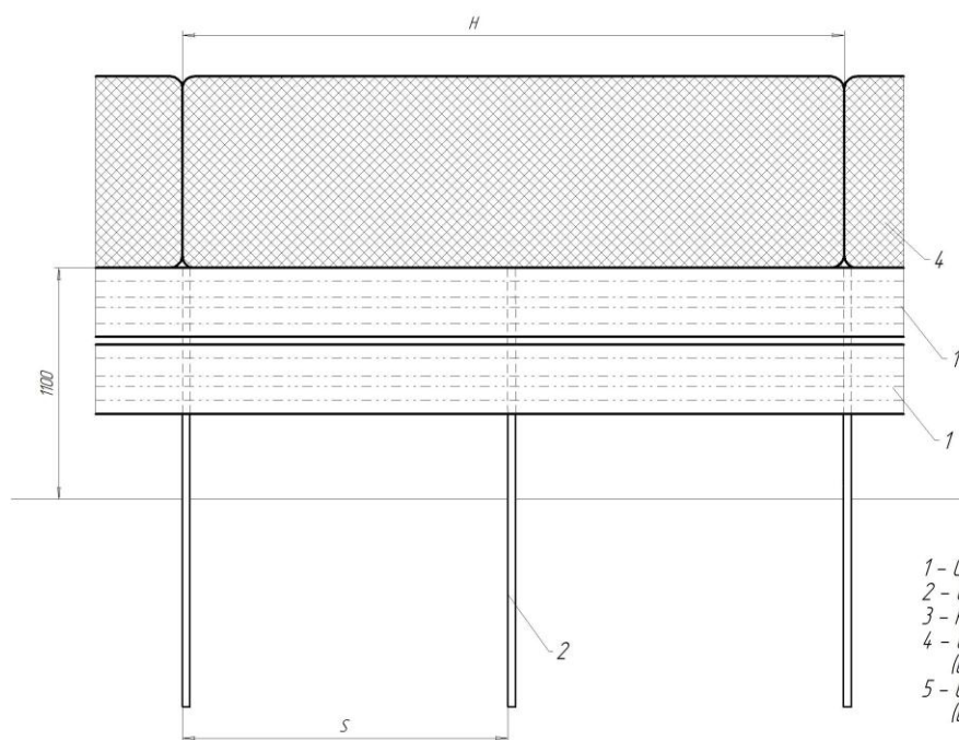
Ограждение с верхней металлической сеткой
