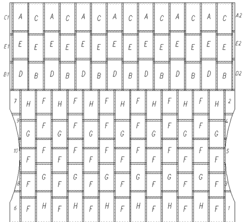
Рисунок 3.1 – Раскладка листов – сборочный чертеж
