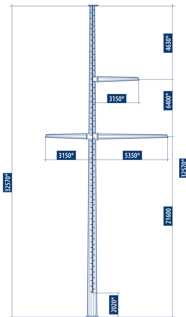
ПРОМЕЖУТОЧНАЯ ОПОРА ПМ220-7Ф
