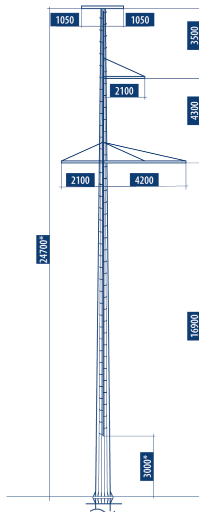
ПРОМЕЖУТОЧНАЯ ОПОРА ПМ110-10Т
