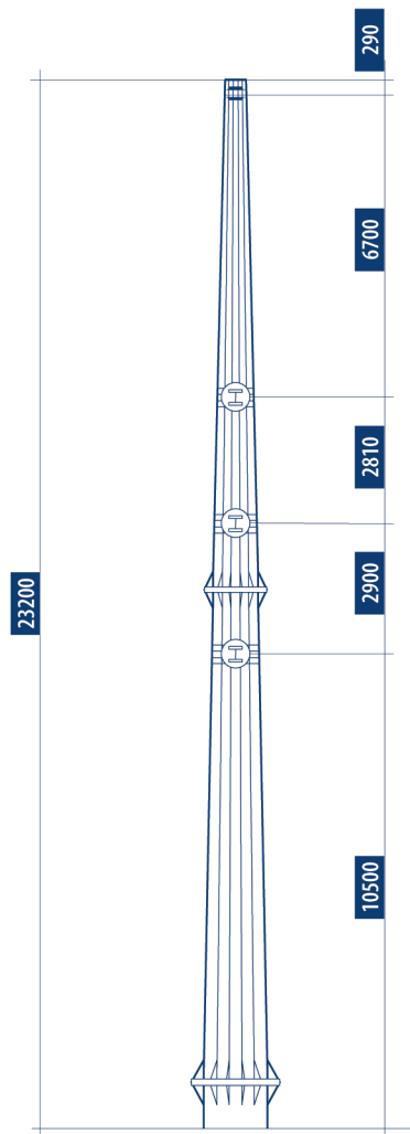
УГЛОВАЯ ОПОРА УМ220-1
