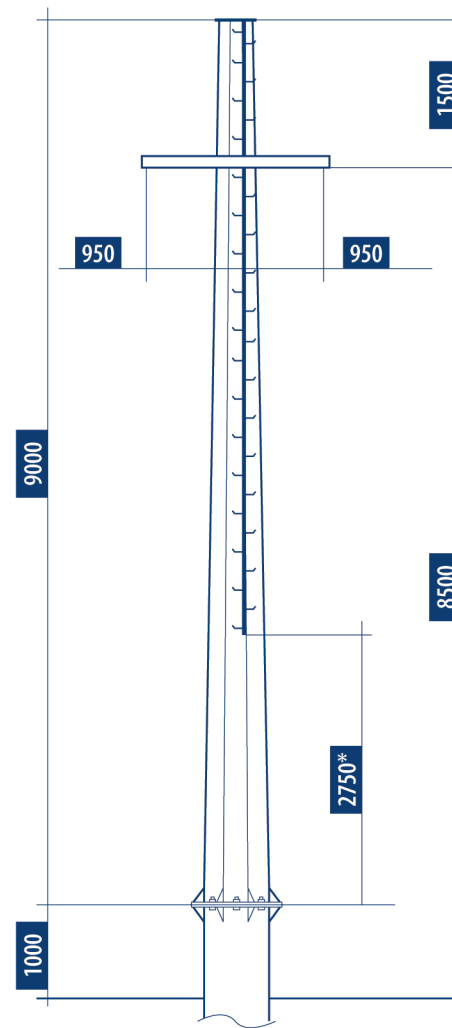
АНКЕРНО-УГЛОВАЯ ОПОРА СМ10АУ
