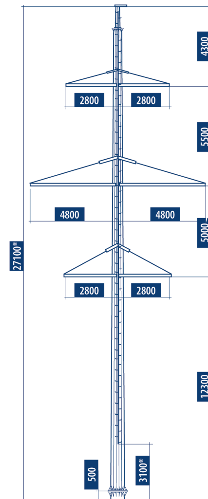
ПРОМЕЖУТОЧНАЯ ОПОРА ПБМ220-2
