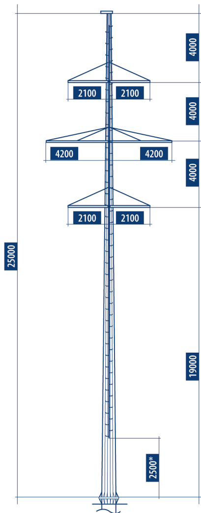
ПРОМЕЖУТОЧНАЯ ОПора ПМ110-4Ф
