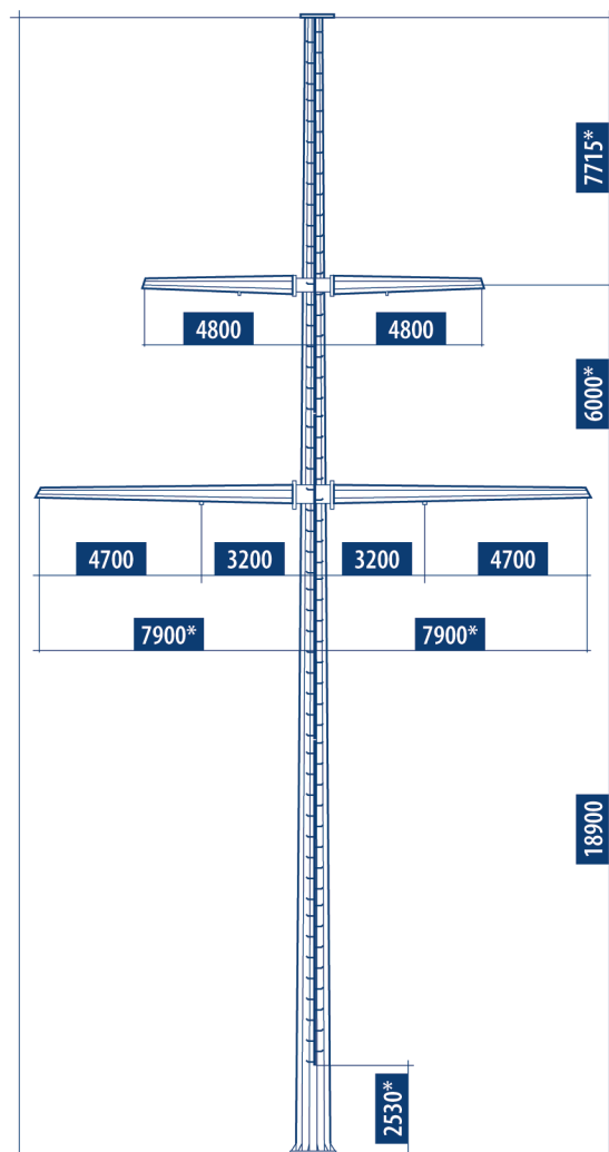
ПРОМЕЖУТОЧНАЯ ОПОРА ПМ220-8Ф
