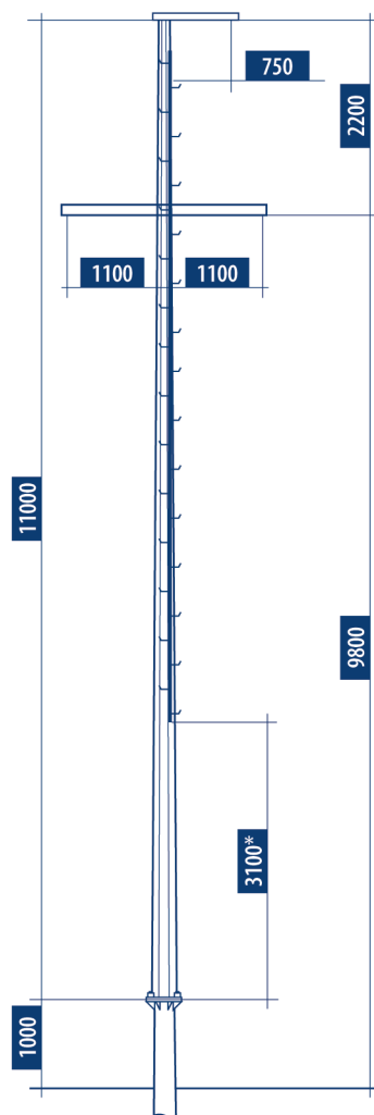
ПРОМЕЖУТОЧНАЯ ОПОРА СМ10П
