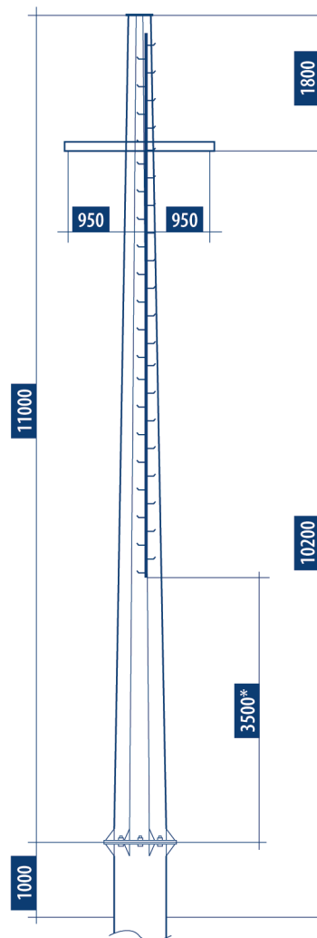
АНКЕРНО-ПЕРЕХОДНАЯ ОПОРА СМ10АП
