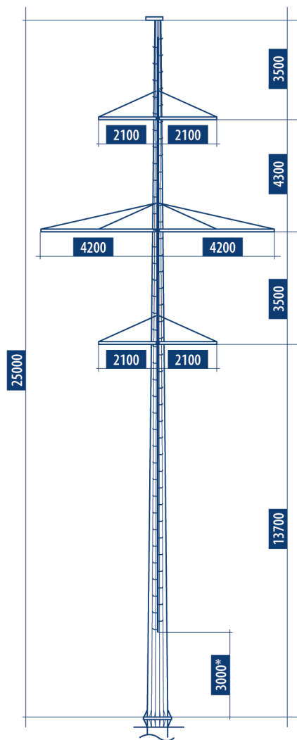
ПРОМЕЖУТОЧНАЯ ОПора ПМ110-2Ф
