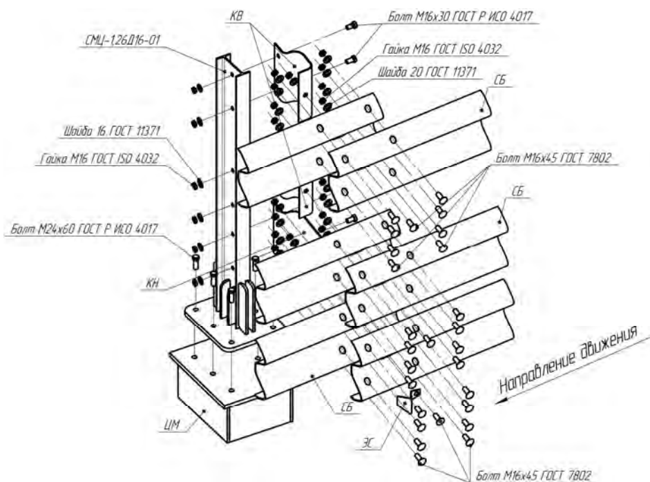
Рисунок В.94 –Схема сборки мостового ограждения 21МО/500÷600-1,5(Ц)xS(Д16)
