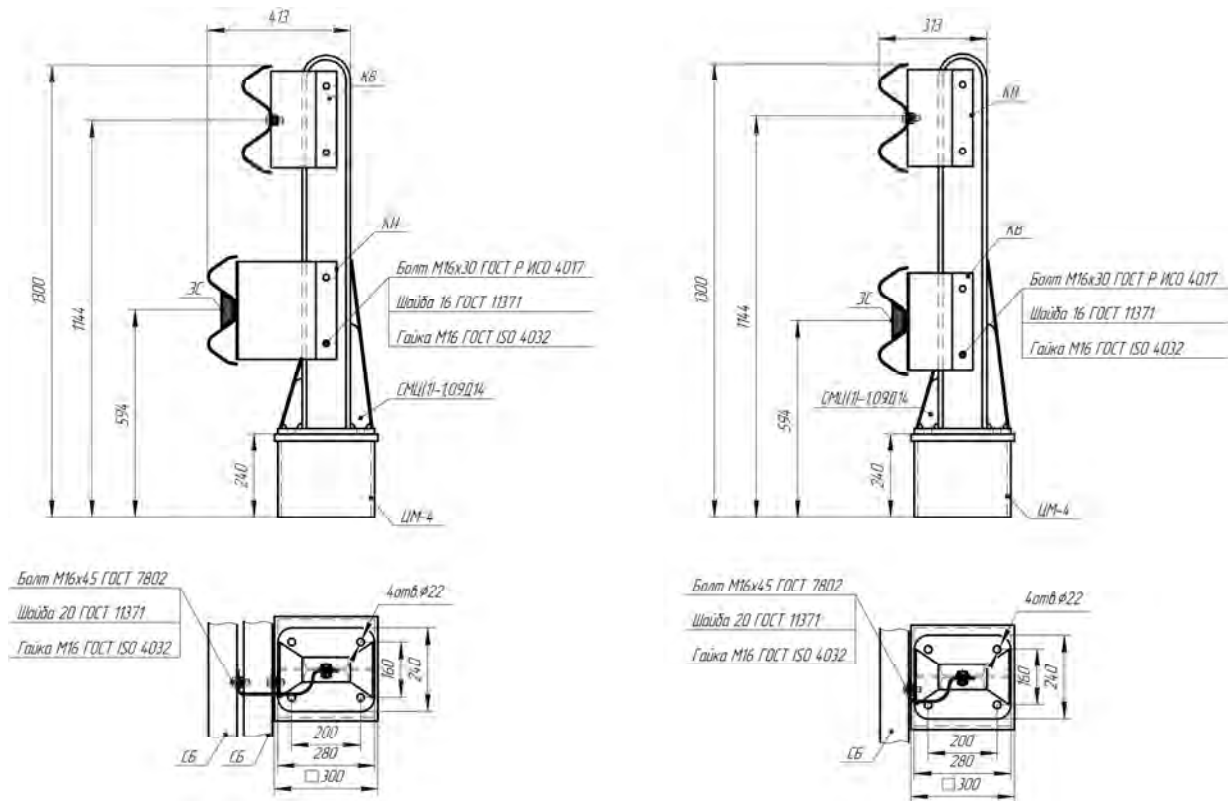
Рисунок В.64- Мостовое ограждение 21МО/500-1,3(Ц)х1,0Д14-0,46(0,85); 21МО/500-1,3(Ц)х1,0Д14-0,46(0,88)
