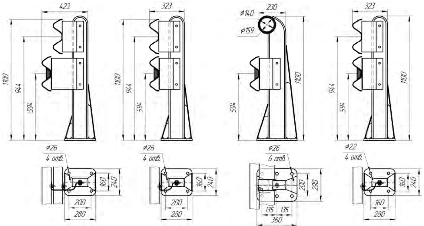
Рисунок 4.30 (СМ(1)-1,1Д16)
