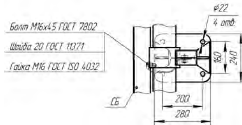
Рисунок В.98 –Мостовое ограждение 21МО/350÷400-0,95(У)хS(Д14)
