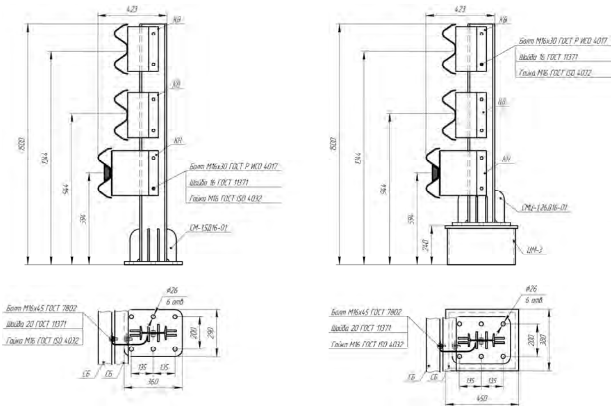
Рисунок В.92 –Мостовое ограждение 21МО/500÷600-1,5xS(Д16); 21МО/500÷600-1,5(Ц)xS(Д16)
