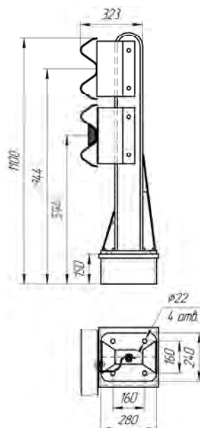
Рисунок 4.68 (СМЦ(2)-0,95Д16) ЦМ-16
