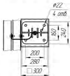
Рисунок 4.51 (СМЦ-0,98Д14) ЦМ-2
