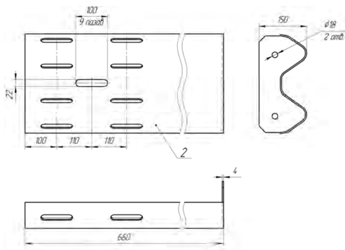
Рисунок Г.9 – Элемент концевой (ЭК-3)
