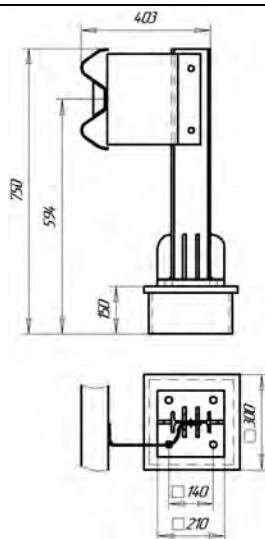
Рисунок 4.8 (СМЦ-0,6Д12) (ЦМ-1)
