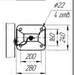
Рисунок 4.29 (СМ(1)-1,33Д14) без КН
