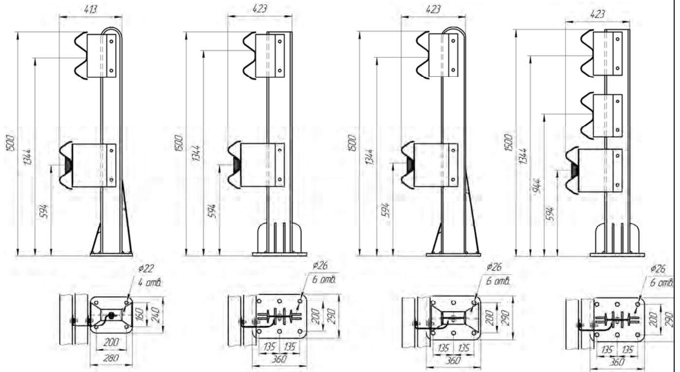
Рисунок 4.38 (СМ(1)-1,53Д14)
