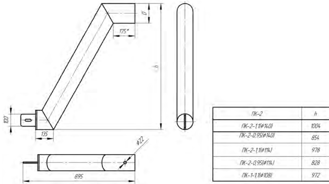
Рисунок Г.13 - Поручень концевой ПК-2
