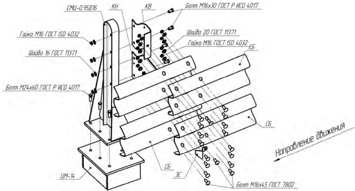
Рисунок В.79 – Схема сборки мостового ограждения 21МО/500÷600-1,1(Ц)
