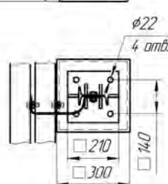
Рисунок 4.56 (СМЦ-0,95Д12) ЦМ-1
