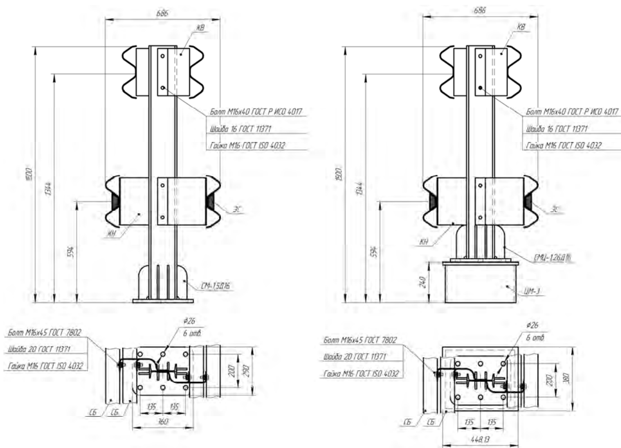
Рисунок В.86 - Мостовое ограждение 21МД/500÷550-1,5xS(Д16); 21МД/500÷550-1,5(Ц)xS(Д16)
