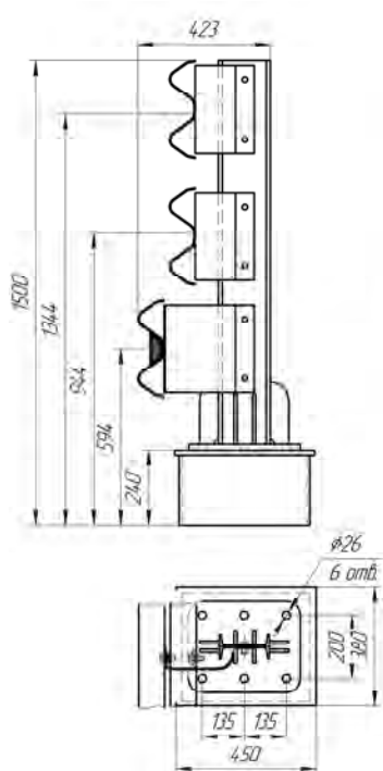
Рисунок 4.65 (СМЦ-1,26Д16-01) ЦМ-3
