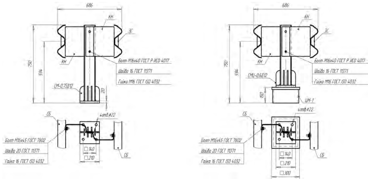
Рисунок В.20 - Мостовое ограждение 21МД/130÷300-0,75xS(Д12); 21МД/130÷300-0,75(П)xS(Д12)
