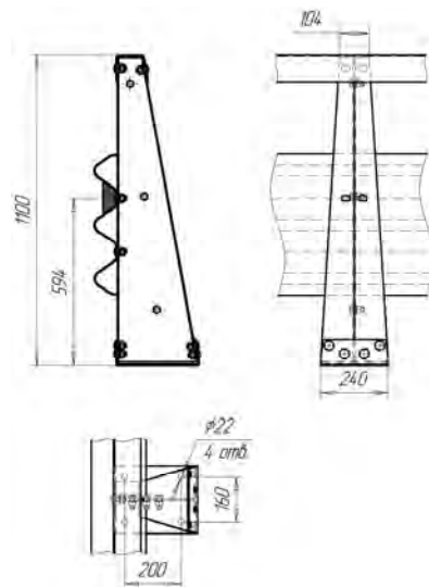
Рисунок 4.42 (СМБ-1,1)
