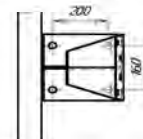
Рисунок 4.5 (СМБ-0,75)
