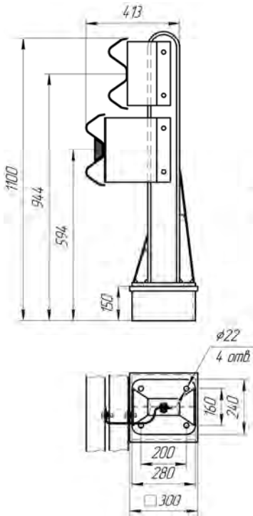
Рисунок 4.58 (СМЦ(1)-0,98Д14) ЦМ-2
