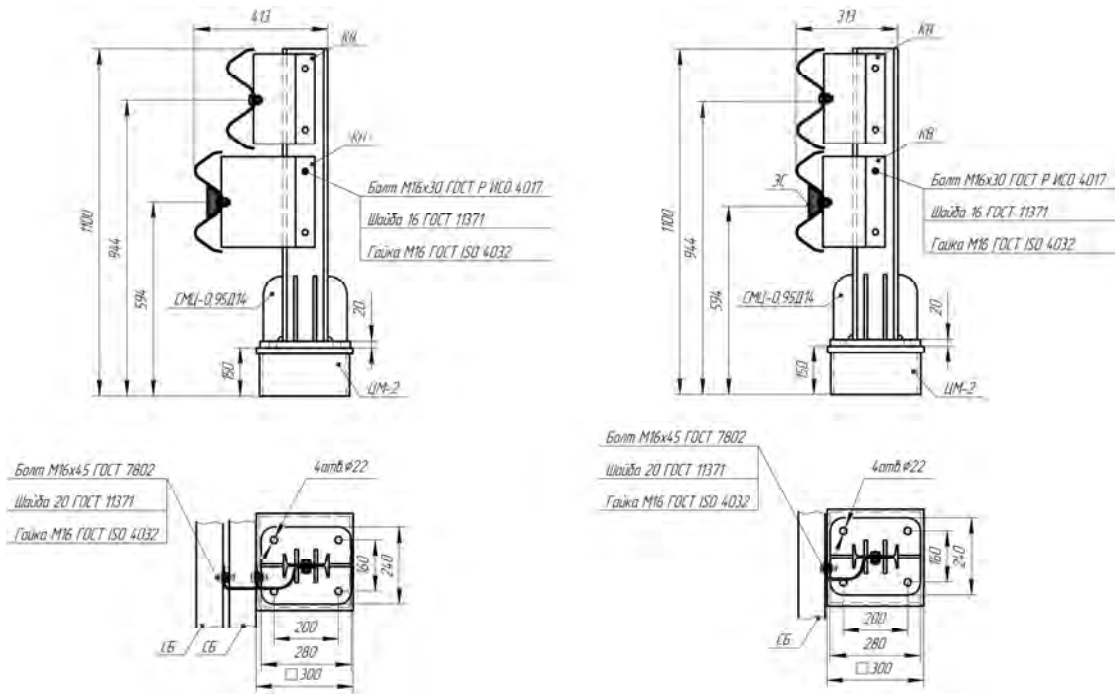
Рисунок В.34 - Ограждение мостовое 21МО/300-450(Д14)Ц; 21МО/300-450(Д14)Ц без КН
