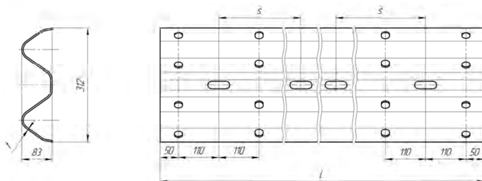
Рисунок Г.2 – Консоль-амортизатор верхний (КВ)
