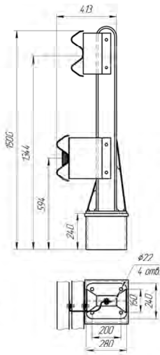
Рисунок 4.67 (СМЦ(1)-1,29Д14) ЦМ-4
