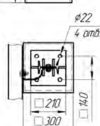
Рисунок 4.57 (СМЦ-0,95Д12) без КН ЦМ-1
