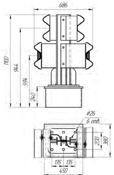
Рисунок 4.83 (СМЦ-0,86Д16) ЦМ-3
