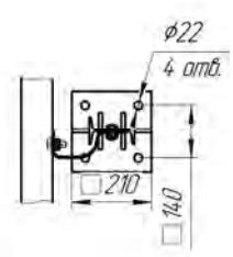
Рисунок 4.21 (СМ-1,1Д12) без КН
