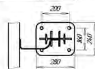
Рисунок 4.3 (СМ-0,75Д14)
