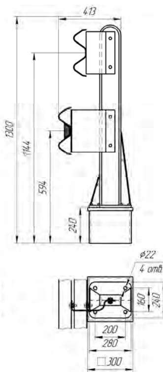
Рисунок 4.71 (СМЦ(1)-1,09Д14) ЦМ-4
