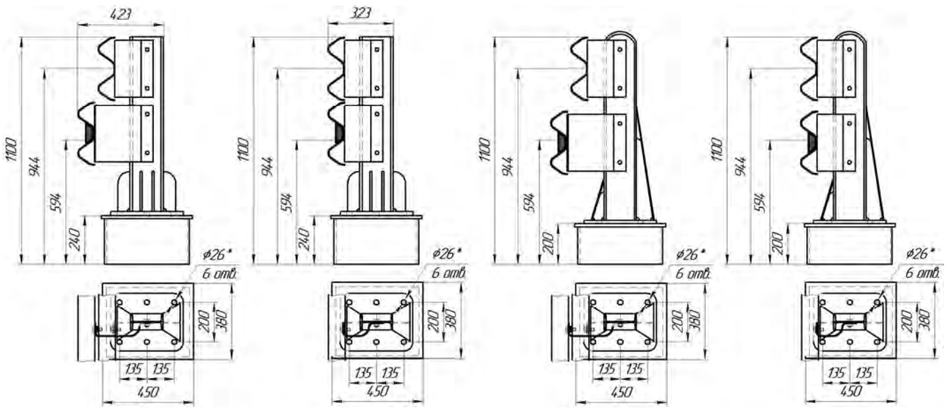
Рисунок 4.73 (СМЦ-0,86Д16) ЦМ-3
