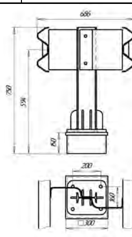
Рисунок 4.13 (СМЦ-0,6Д14) (ЦМ-2)
