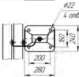
Рисунок 4.26 (СМ(1)-1,13Д14)
