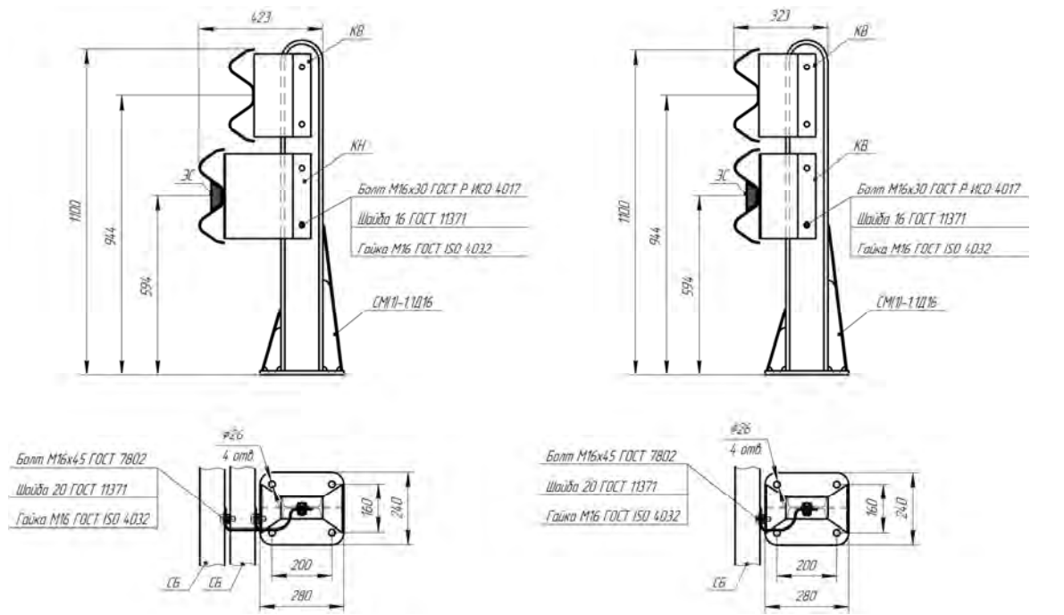
Рисунок В.56 - Мостовое ограждение 21МО/350÷450-1,1xS(Д16); 21МО/350÷450-1,1xS(Д16) без КН
