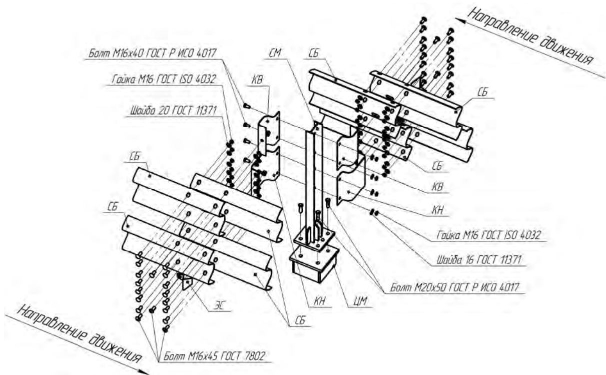
Рисунок В.40 – Схема сборки мостового ограждения 21МД/300÷450-1,1(Ц)
