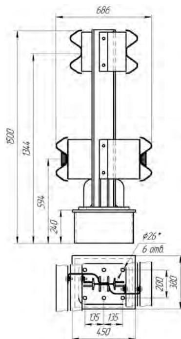
Рисунок 4.84 (СМЦ-1,26Д16) ЦМ-15
