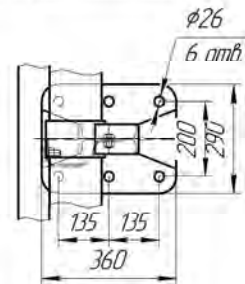
Рисунок 4.23 (СМУ-0,95Д16)
