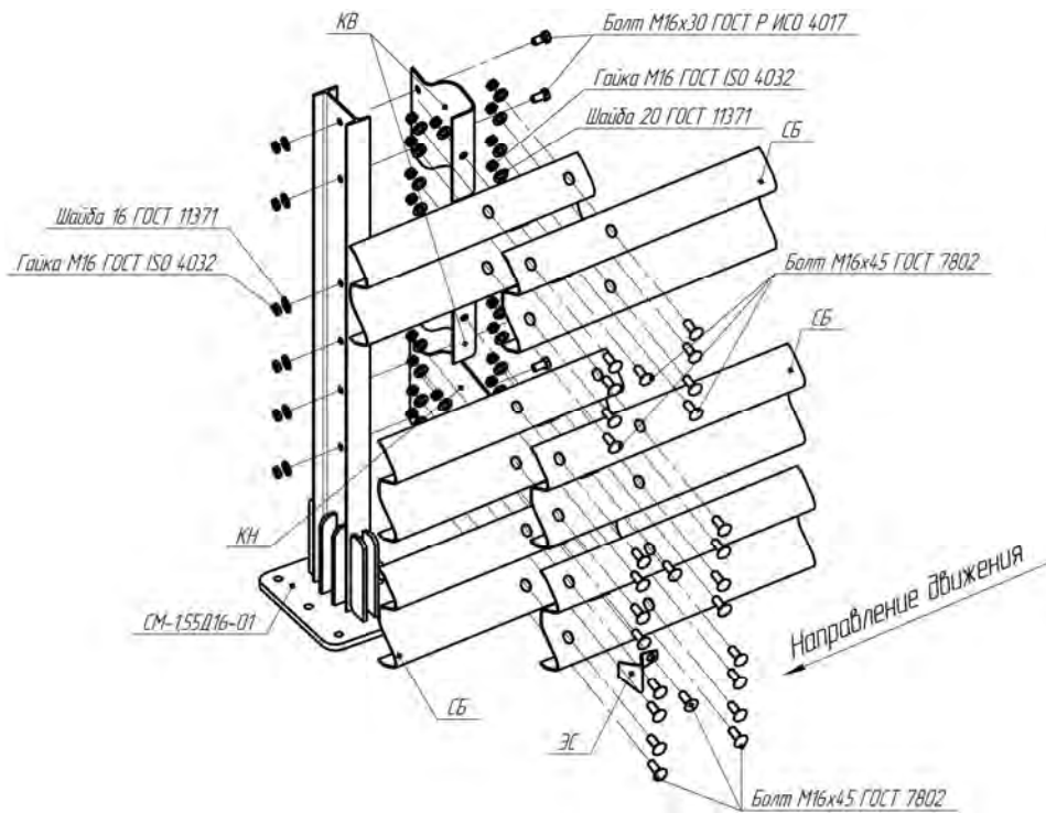
Рисунок В.93 –Схема сборки мостового ограждения 21МО/500÷600-1,5xS(Д16)
