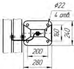
Рисунок 4.18 (СМ(1)-0,93Д14)
