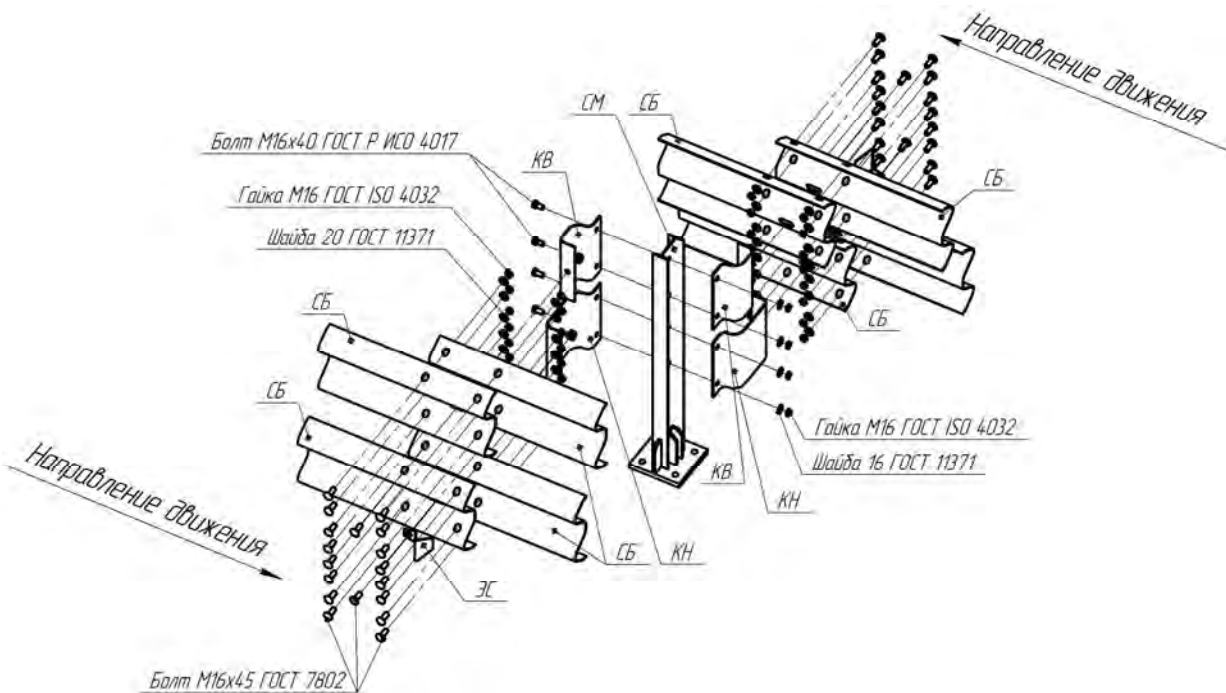
Рисунок В.39 – Схема сборки мостового ограждения 21МД/300÷450-1,1(Д14)
