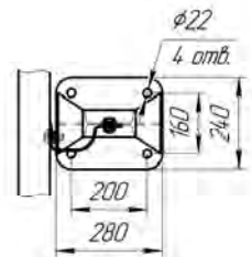
Рисунок 4.19 (СМ(1)-0,93Д14) без КН
