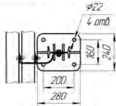
Рисунок 4.14 (СМ-1,1Д14)
