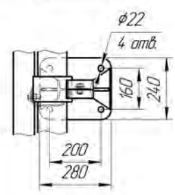
Рисунок 4.25 (СМУ-1,1Д14)
