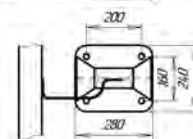
Рисунок 4.4 (СМ(1)-0,78Д14)
