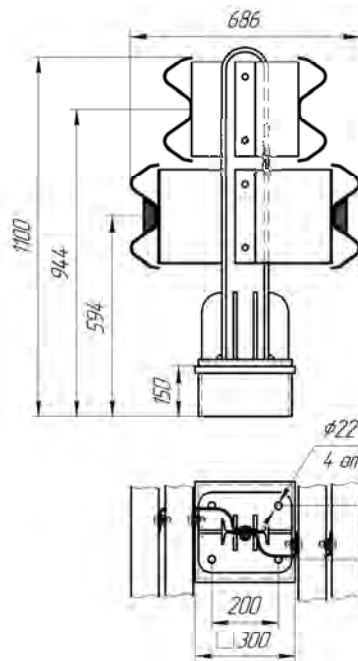
Рисунок 4.82 (СМЦ-0,98Д14) ЦМ-2
