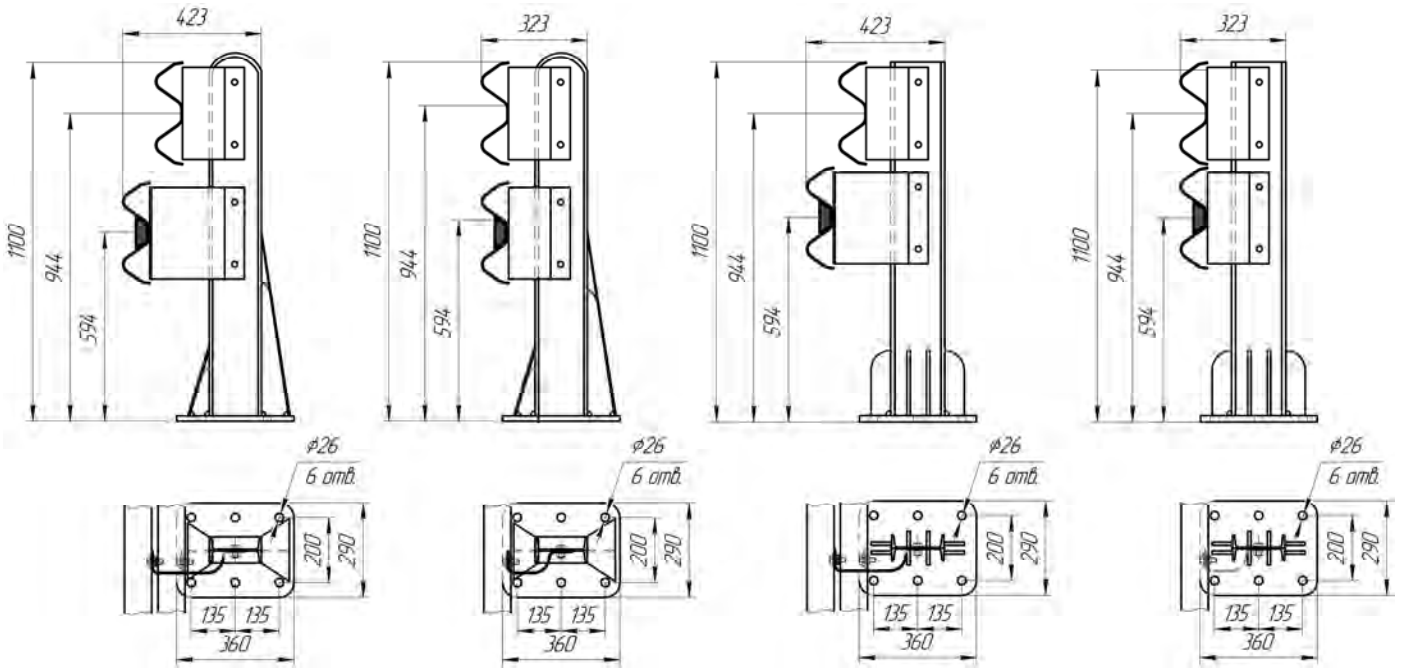
Рисунок 4.34 (СМ-1,15Д16)
