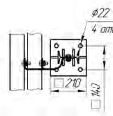
Рисунок 4.20 (СМ-1,1Д12)
