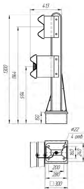
Рисунок 4.69 (СМЦ(1)-1,18Д14) ЦМ-2
