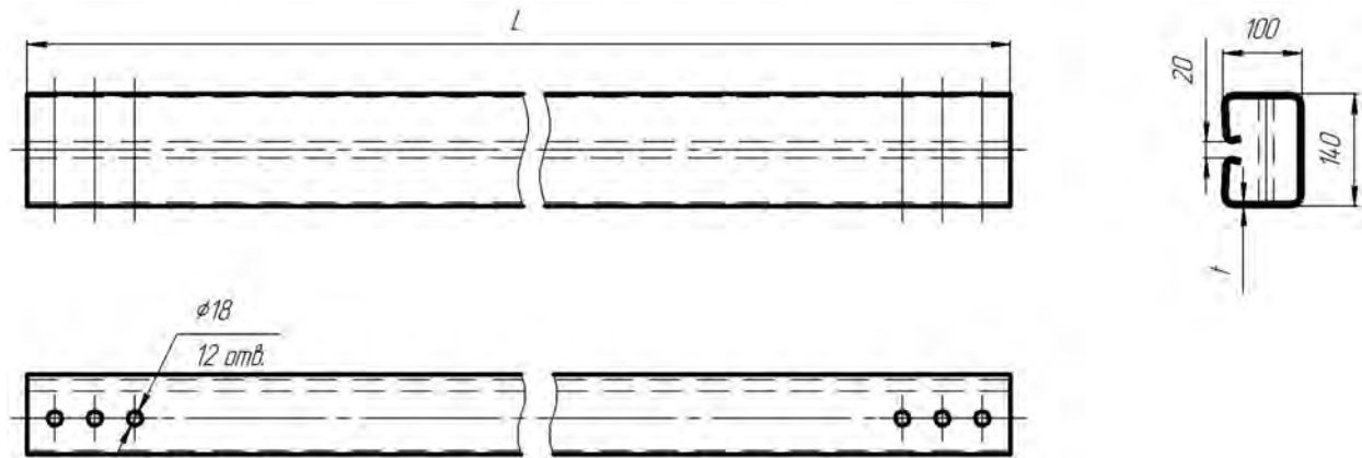
Рисунок Г.15 –Секция балки СБ-Б1 коробчатого профиля
