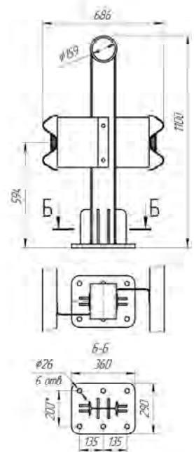
Рисунок 4.49 (СМДУ-1,1Д16)
