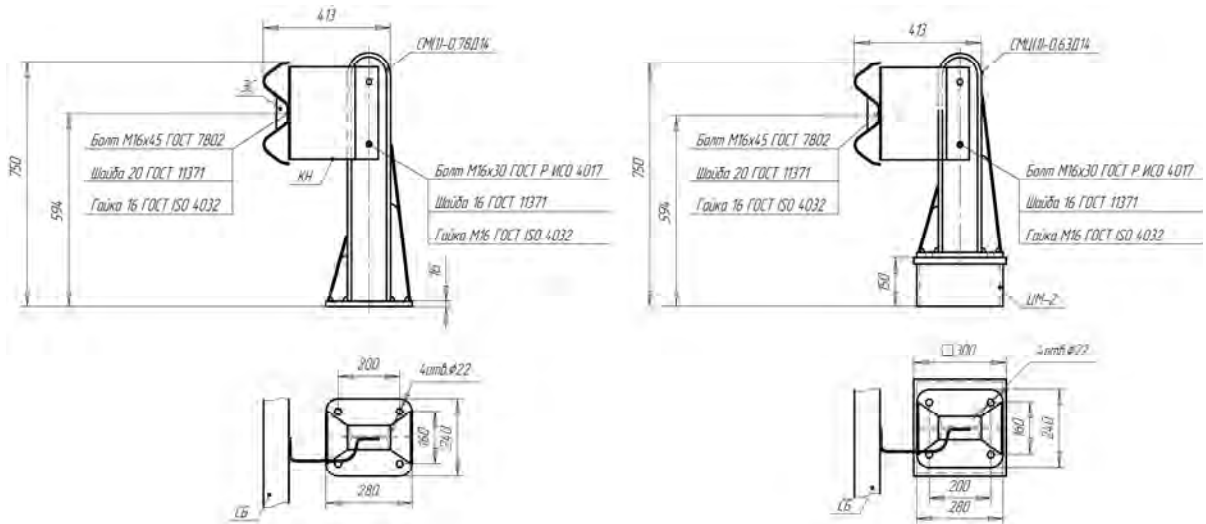
Рисунок В.17 - Мостовое ограждение 21МО/130÷300-0,75xS(Д14); 21МО/130÷300-0,75(Ц)xS(Д14)
