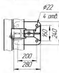
Рисунок 4.24 (СМУ-1,1Д14(127))
