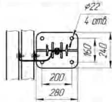
Рисунок 4.15 (СМ-1,13Д14)
