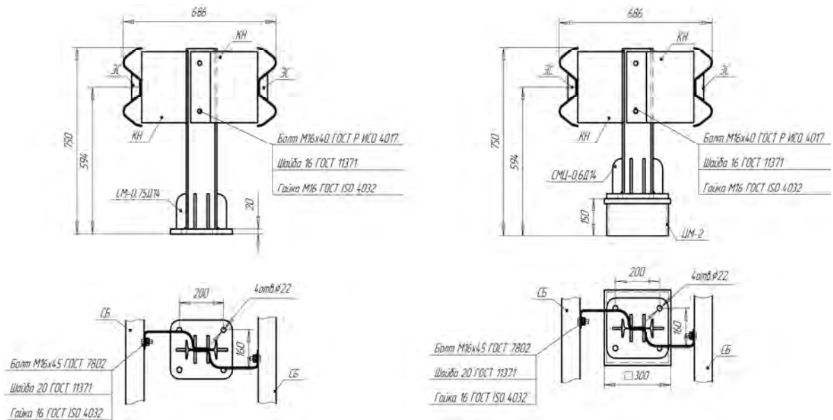
Рисунок В.21 - Мостовое ограждение на поколе 21МД/130÷300-0,75xS(Д14); 21МД/130÷300-0,75(П)xS(Д14)
