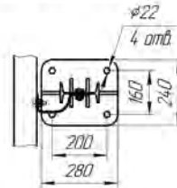
Рисунок 4.16 (СМ-1,1Д14) без КН
