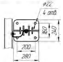
Рисунок 4.17 (СМ-1,13Д14) без КН
