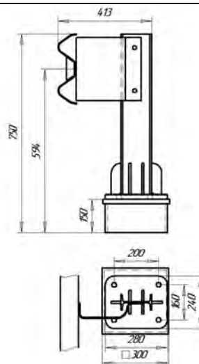
Рисунок 4.9 (СМЦ-0,6Д14) (ЦМ-2)
