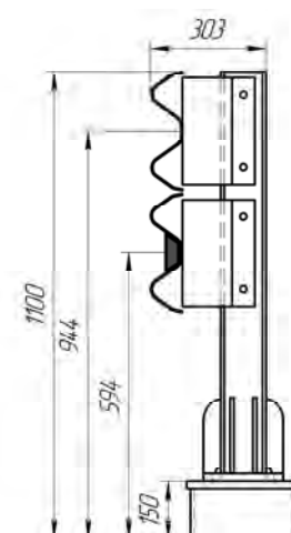
Рисунок 4.53 (СМЦ-0,98Д14) без КН ЦМ-2
