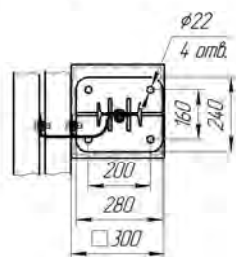
Рисунок 4.50 (СМЦ-0,95Д14) ЦМ-2
