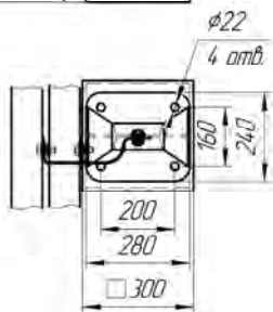
Рисунок 4.54 (СМЦ(1)-0,78Д14) ЦМ-2
