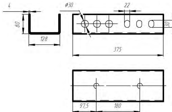
Рисунок Г.16 – Основные параметры вставки В-1
