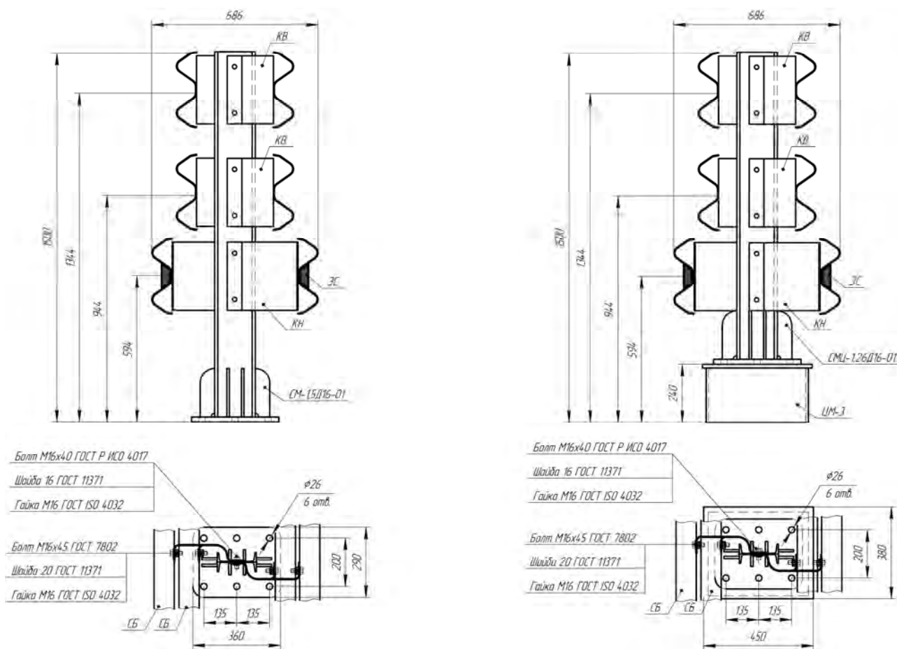
Рисунок В.95 –Мостовое ограждение 21МД/500÷600-1,5xS(Д16); 21МО/500÷600-1,5(Ц)xS(Д16)
