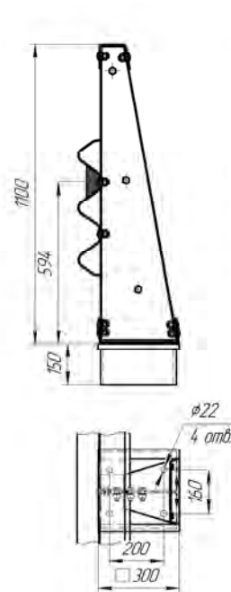
Рисунок 4.64 СМБ(II)-0,95 ЦМ-2
