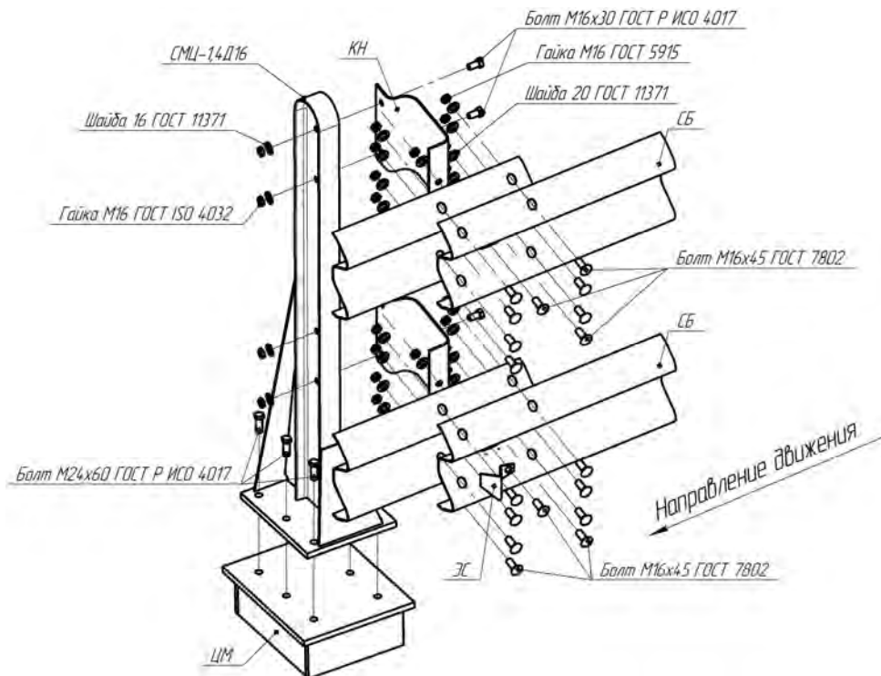
Рисунок В.91 – Схема сборки мостового ограждения 21МО/600-1,5(Ц)x2,0Д16-0,59(0,68)
