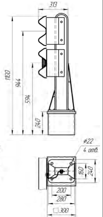
Рисунок 4.61 (СМЦ(1)-0,89Д14) без КН ЦМ-4
