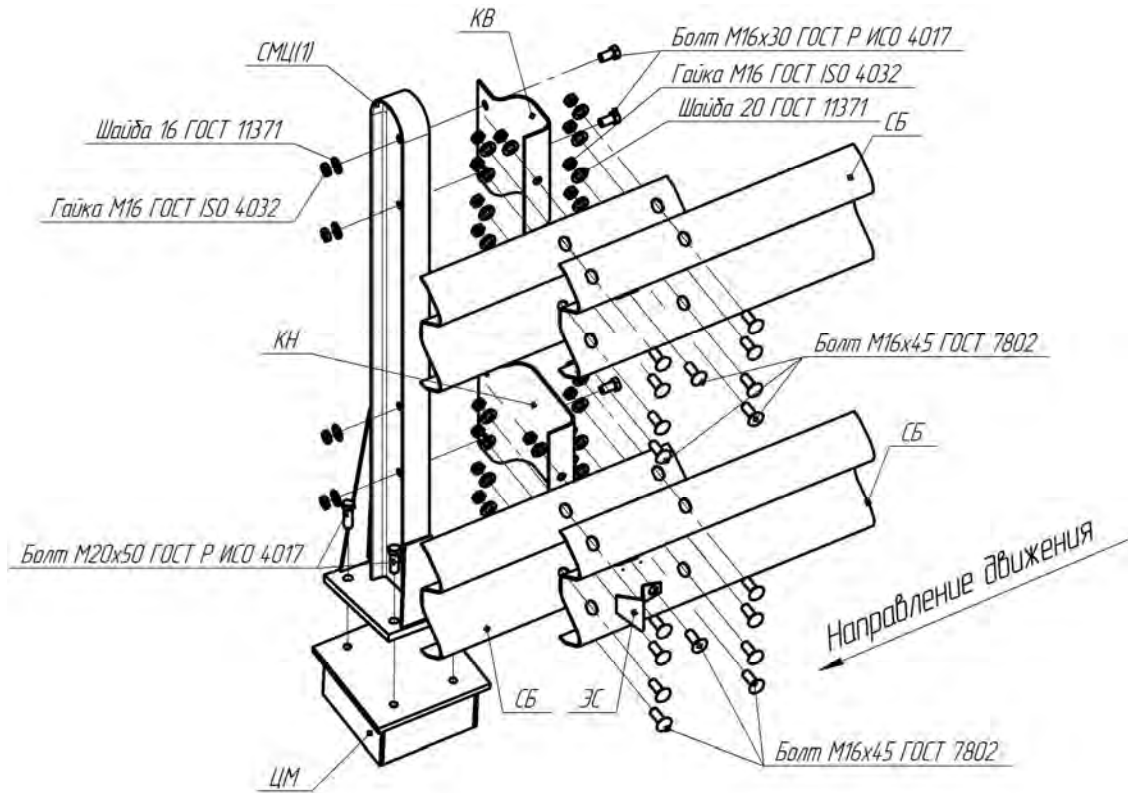
Рисунок В.66 – Схема сборки мостового ограждения 21МО/500-1,3(Ц)
