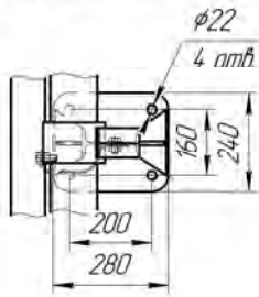
Рисунок 4.22 (СМУ-0,95Д14)
