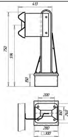
Рисунок 4.10 (СМЦ(1)-0,63Д14) (ЦМ-2)
