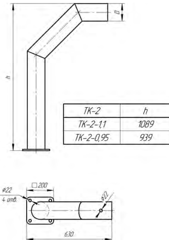
Рисунок Г.14 – Труба усиления концевая (ТК-2)
