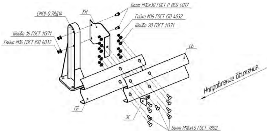
Рисунок В.18 – Схема сборки мостового ограждения 21МО/130÷300-0,75
