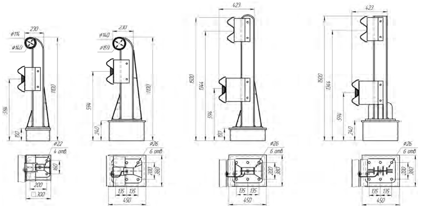
Рисунок 4.77 (СМУ(Ц)-0,95Д14) ЦМ-2
