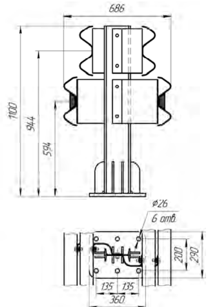
Рисунок 4.45 (СМ-1,1Д16)
