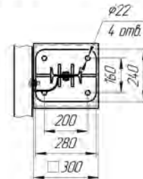
Рисунок 4.53 (СМЦ-0,98Д14) без КН ЦМ-2
