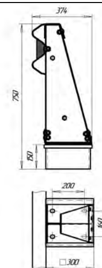
Рисунок 4.11 (СМБ(Ц)) (ЦМ-2)
