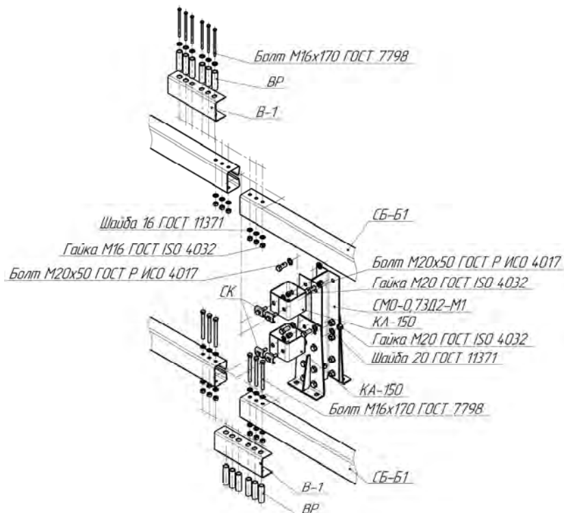
Рисунок В.19.1 – Мостовое ограждение 21МО/300-0,75х2,0Д-М1
