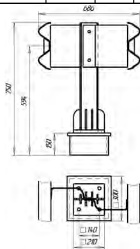
Рисунок 4.12 (СМЦ-0,6Д12) (ЦМ-1)
