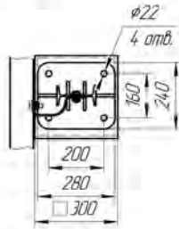
Рисунок 4.52 (СМЦ-0,95Д16) без КН ЦМ-2
