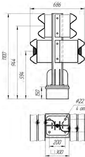
Рисунок 4.81 (СМЦ-0,95Д14) ЦМ-2
