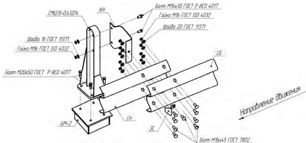
Рисунок В.19 – Схема сборки мостового ограждения на цоколе
