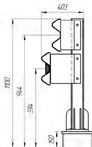
Рисунок 4.52 (СМЦ-0,95Д16) без КН ЦМ-2
