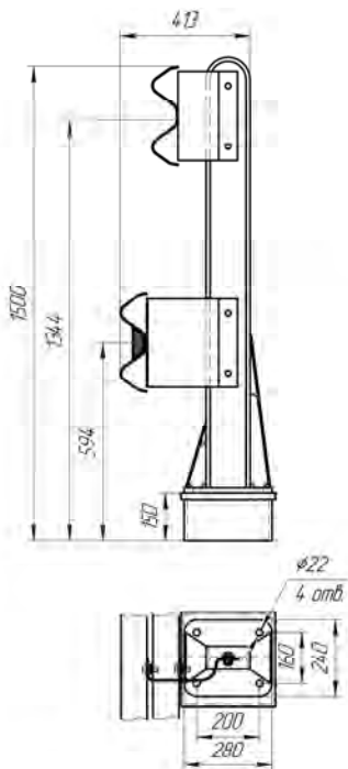
Рисунок 4.66 (СМЦ(1)-1,38Д14) ЦМ-2
