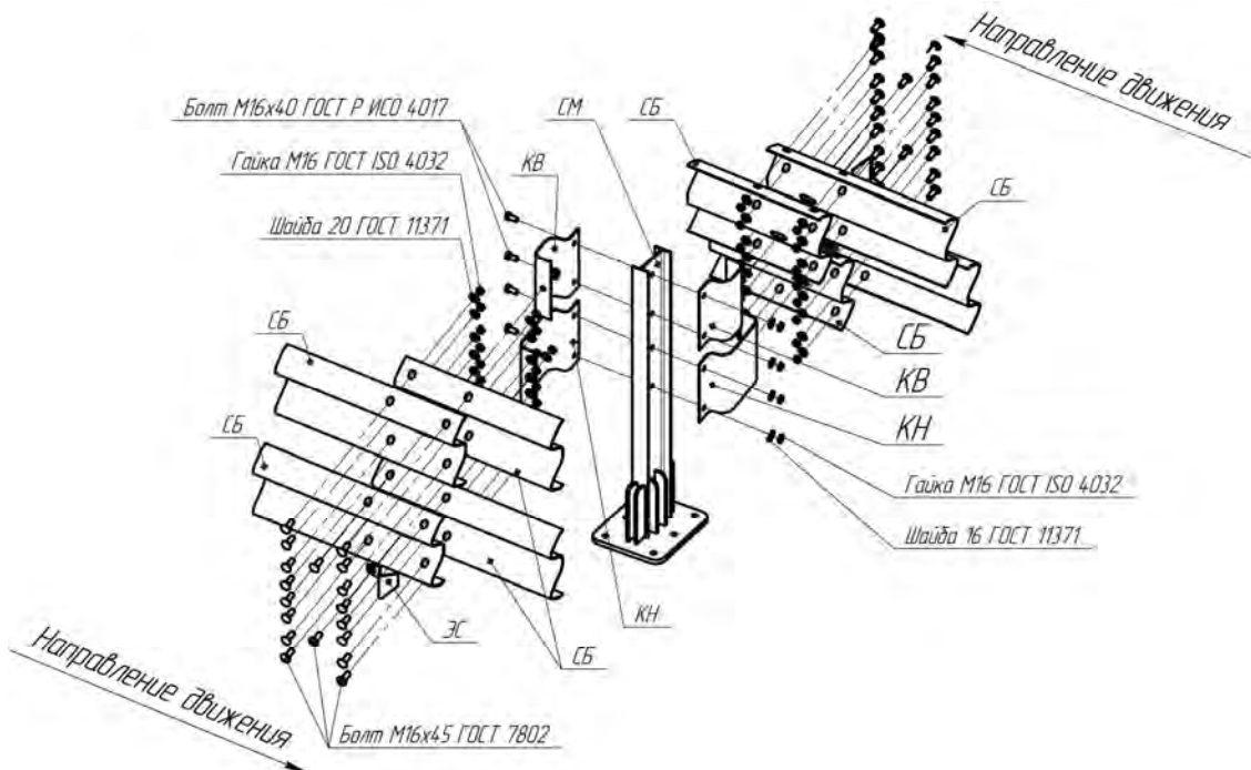
Рисунок В.74 – Схема сборки мостового ограждения 21МД/500÷550-1,1
