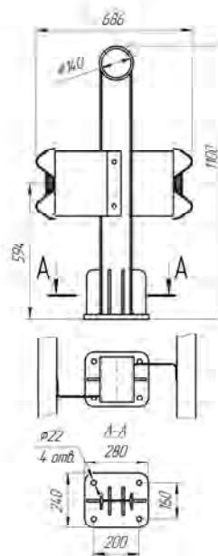
Рисунок 4.48 (СМДУ-1,1Д14)
