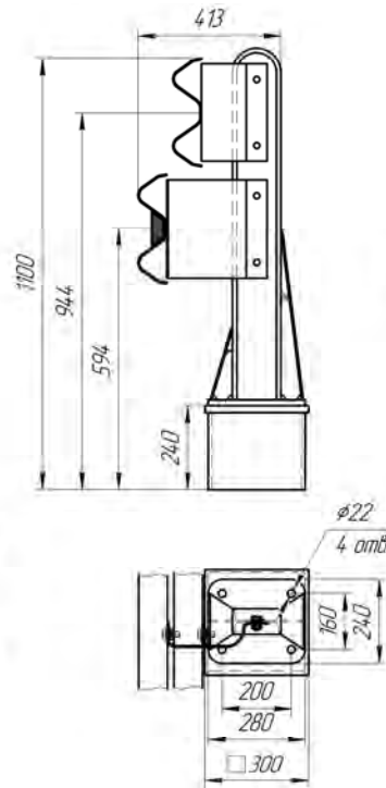
Рисунок 4.60 (СМЦ(1)-0,89Д14) ЦМ-4
