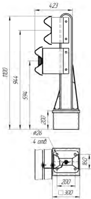
Рисунок 4.62 (СМЦ(1)-0,95Д16) ЦМ-13
