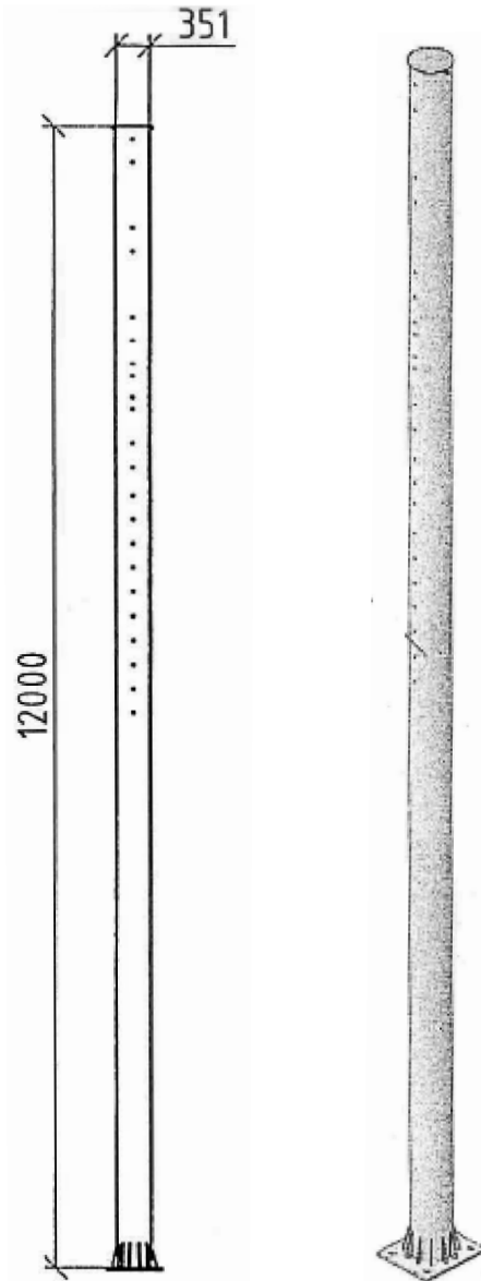
МТК Стойки металлические консольные кольцевого сечения высотой 12,0 метров
